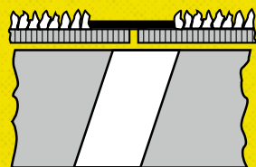
Шов 6 G Косой срез. Стыковое соединение, подклеенное армированной пленкой со стороны зерен. В месте соедине- ния зерно полностью сошлифовано. Используется на оборудовании с плоскими контактными элементами
