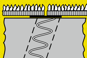
Шов 3 G Зигзагообразное соединение упроч- ненное пленкой. Обеспечивает спо- койный ход без биения, для обработки хрупких элементов, особенно стекла
