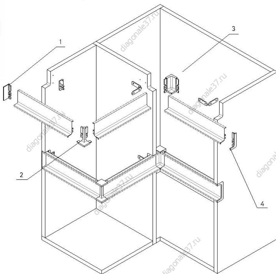
Схема сборки
