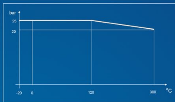
Diagramm: Druck/Temperatur
