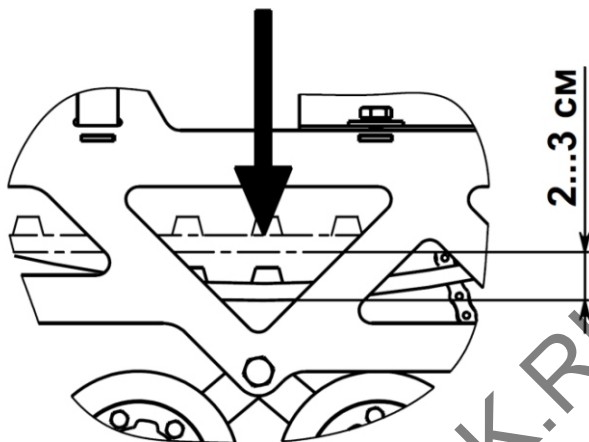
Рис.6 Проверка натяжения гусеницы
