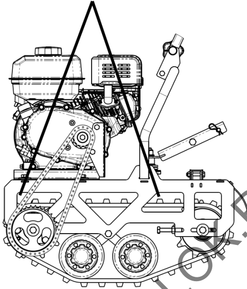
Рис.9 Схема строповки мотобуксировщика при погрузке
