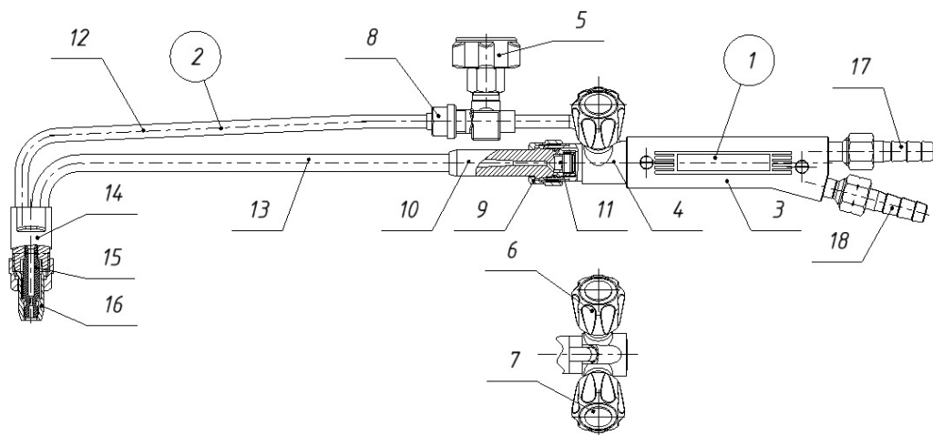
Рис. 1- ствол, 2- наконечник, 3- рукоятка, 4- корпус, 5- вентиль режущего кислорода, 6- вентиль подогревающего кислорода, 7- вентиль горючего газа, 8, 9- накидные гайки, 10- смесительная камера, 11- инжектор, 12, 13- соединительные трубки, 14- головка резака, 15- сменный внутренний мундштук, 16- сменный наружный мундштук, 17, 18- ниппели.
