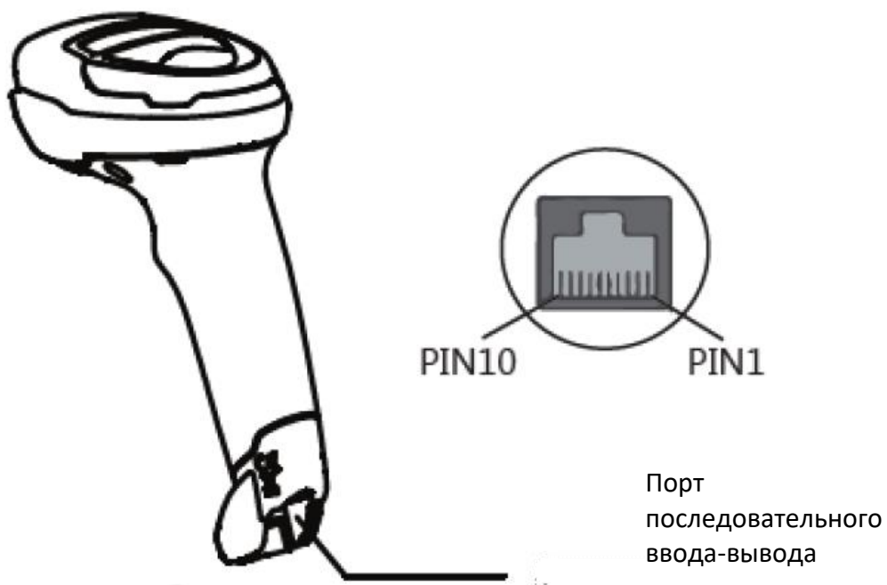
Рисунок 2. Расположение порта последовательного ввода-вывода
