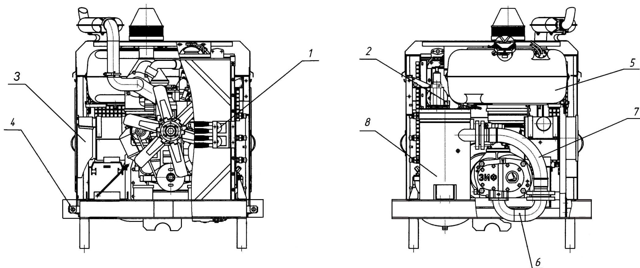
1 – масляный радиатор; 2 – фильтр линии отсоса; 3 – ящик ЗИП; 4 – шкворневые запоры; 5 – бак топливный; 6 – труба нагнетания; 7 – сильфонная труба; 8 – маслоотделитель;
