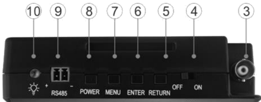
Рис. 4 Fiesta T-2, разъемы, кнопки и индикаторы на верхней панели
