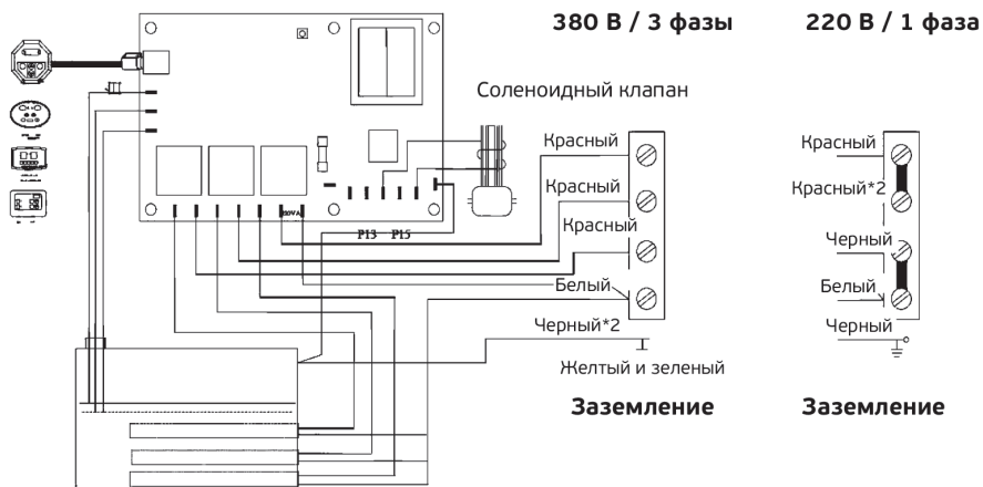
Рисунок 1. Схема подключения парогенератора
