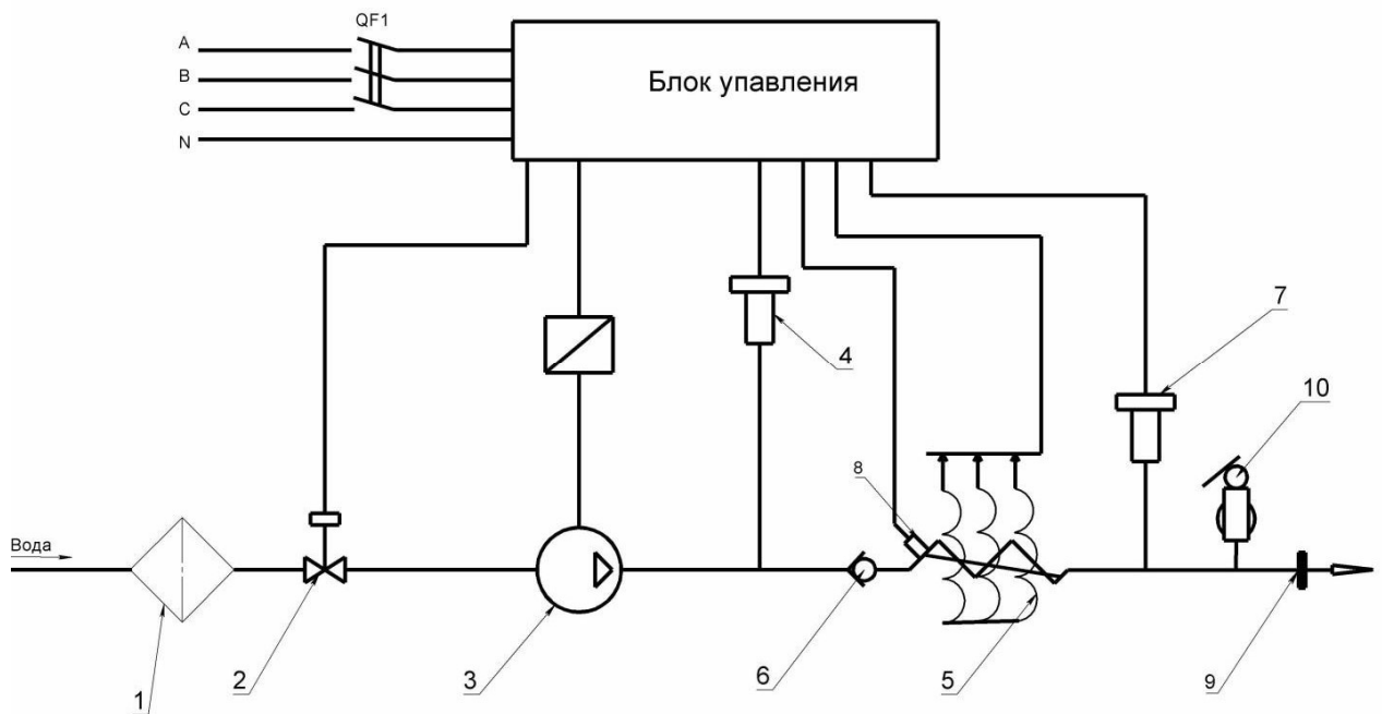
Рис.2. Принципиальная электрогидравлическая схема парогенератора
