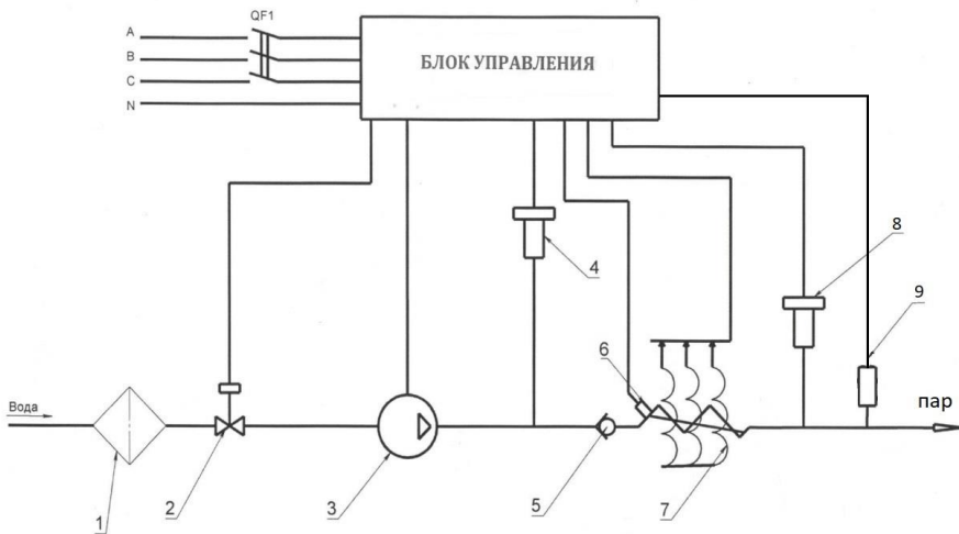
Рис.2. Принципиальная электрогидравлическая схема парогенератора
