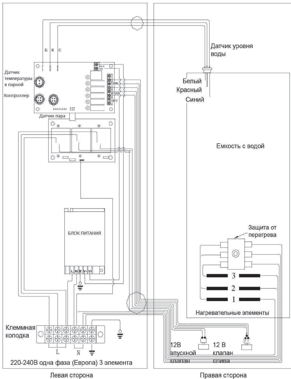
Рисунок 10. Электромонтажная схема TOLO-40 KEY - TOLO-80 KEY
