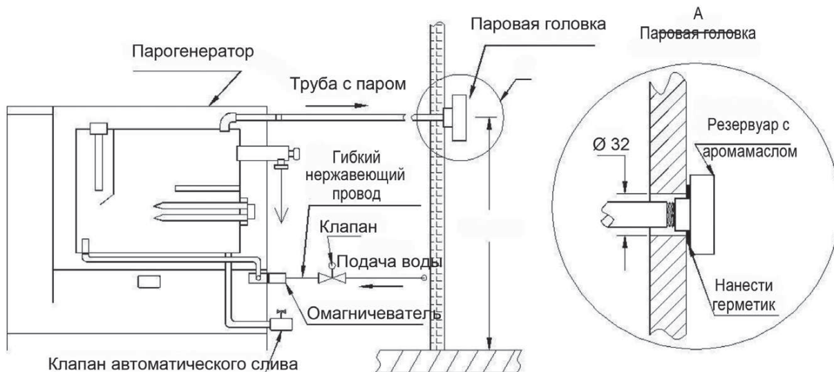
Рисунок 7. Схема установки труб
