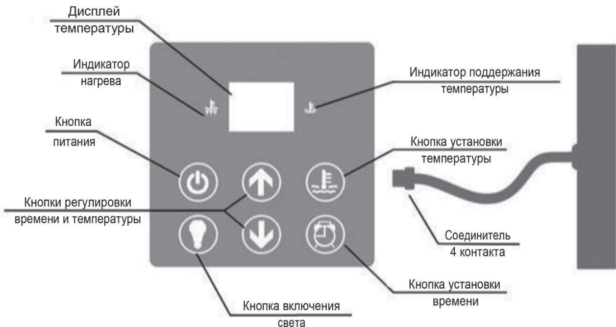
Рисунок 3. Панель управления
