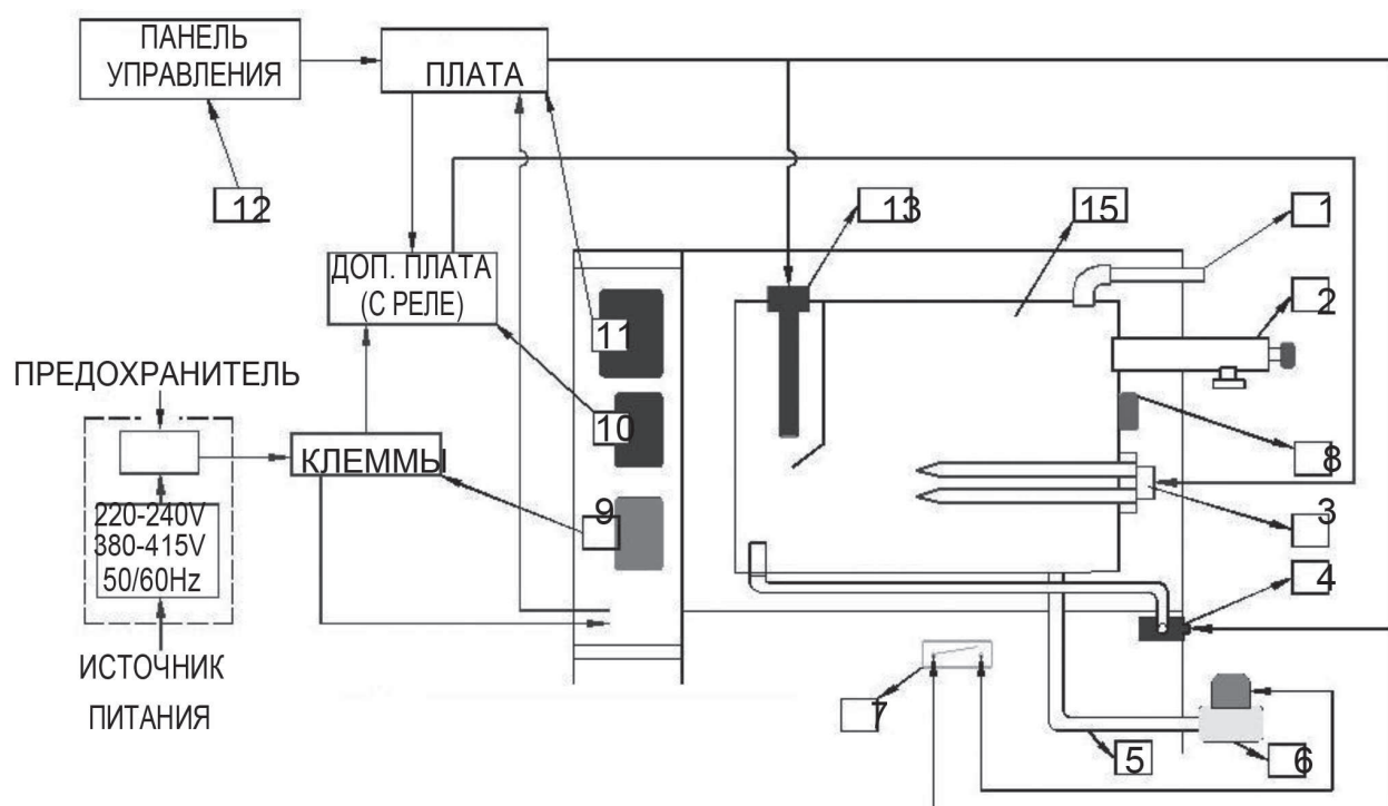
Рисунок 2. Принцип работы парогенератора
