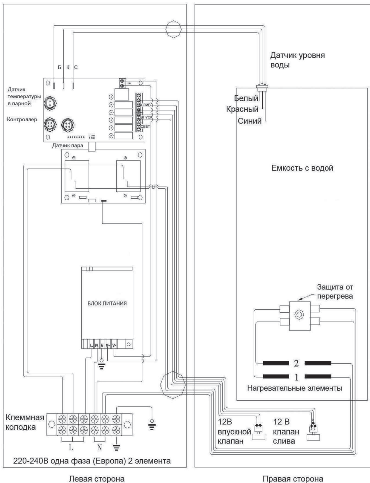
Рисунок 9. Электромонтажная схема TOLO-30 KEY
