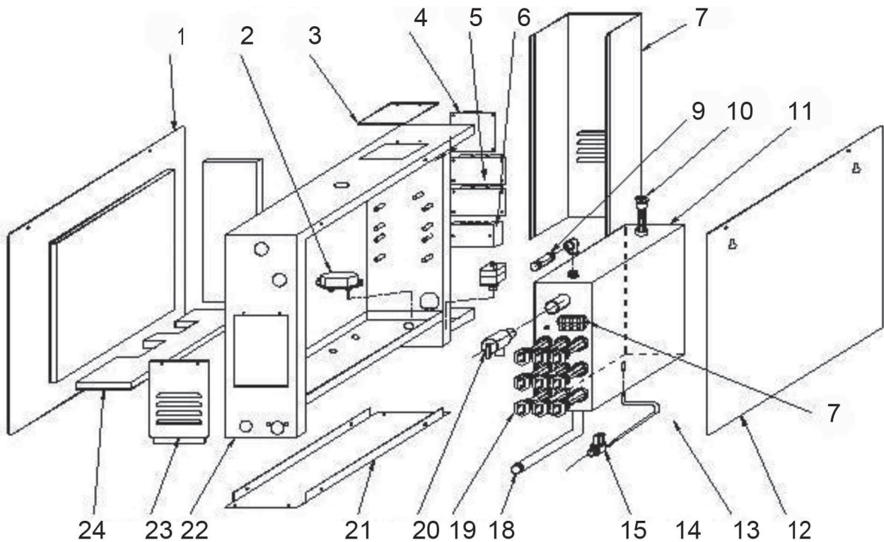
Рисунок 1. Конструкция парогенератора
