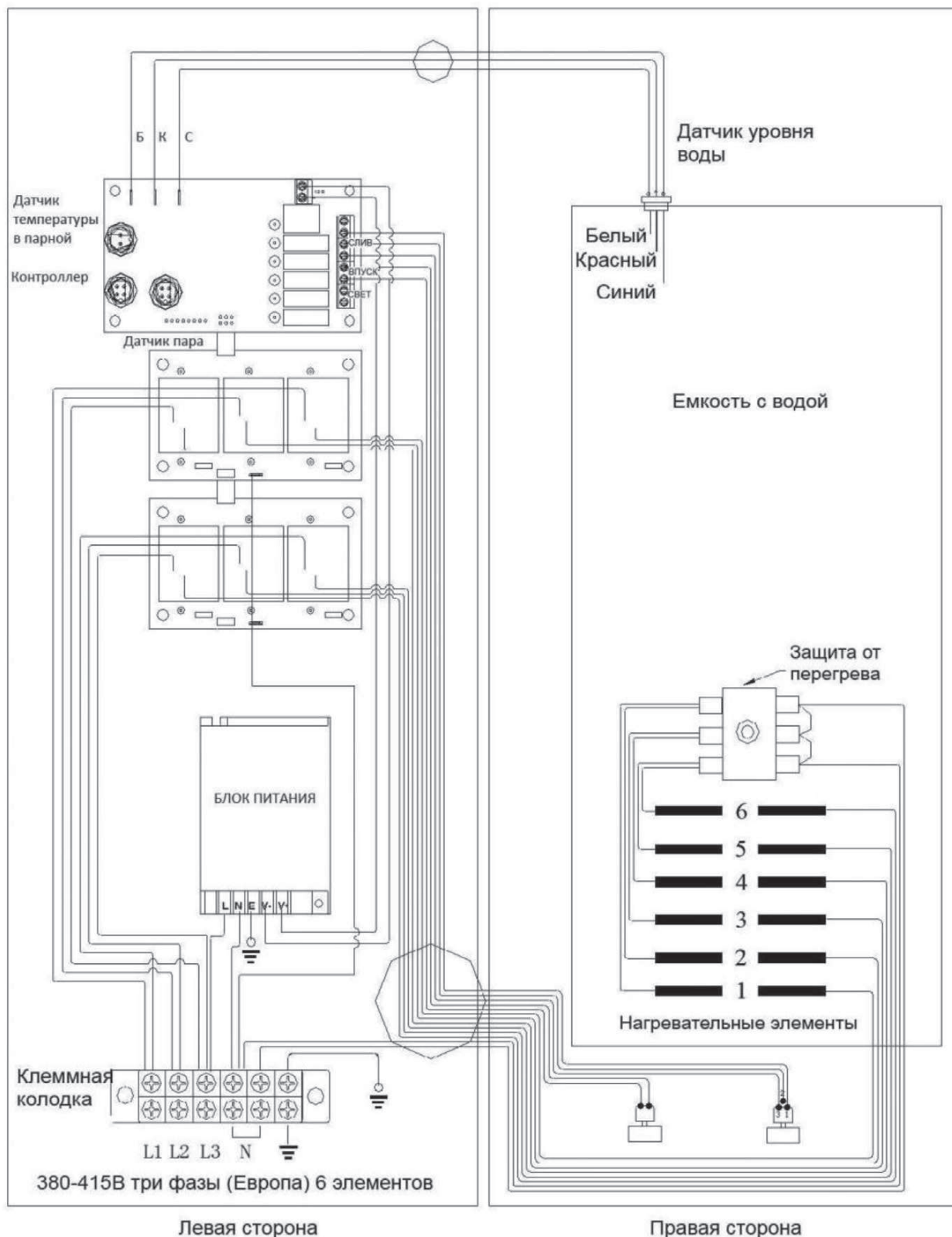
Рисунок 11. Электромонтажная схема TOLO-90 KEY - TOLO-135 KEY
