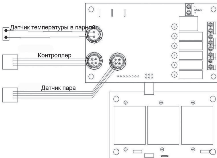
Рисунок 8. Схема подключения электропитания
