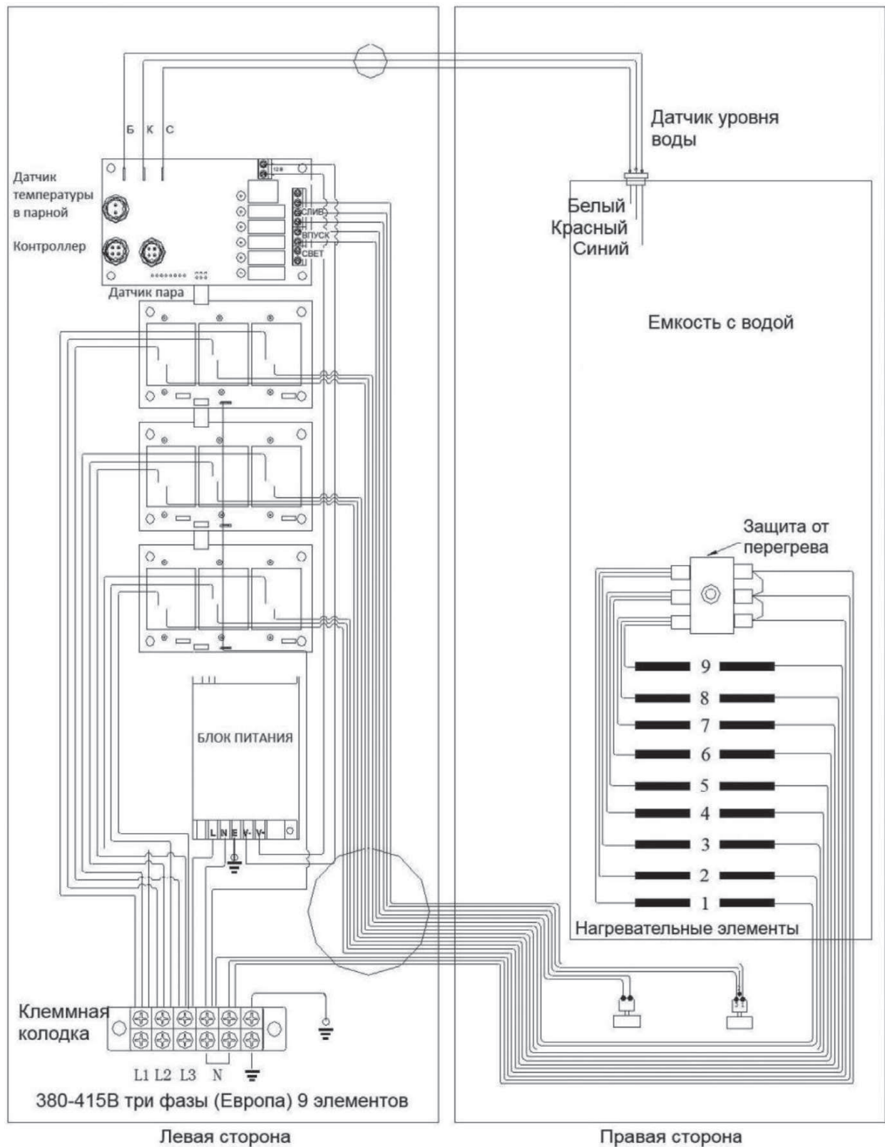
Рисунок 12. Электромонтажная схема TOLO-150 KEY - TOLO-240 KEY
