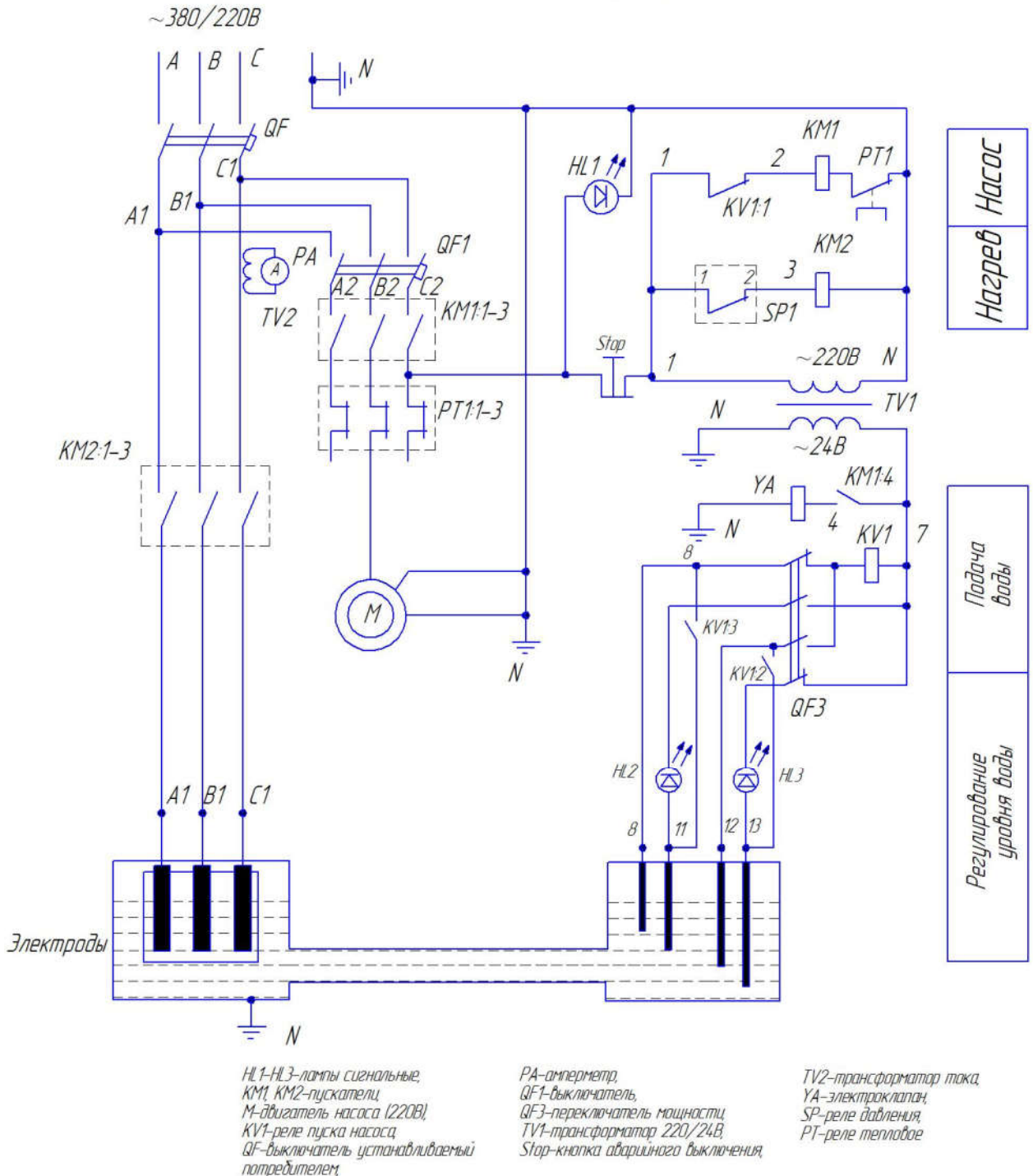
Рис.10 Схема электрическая двухступенчатых парогенераторов (управление тока нагрева пускателем)
