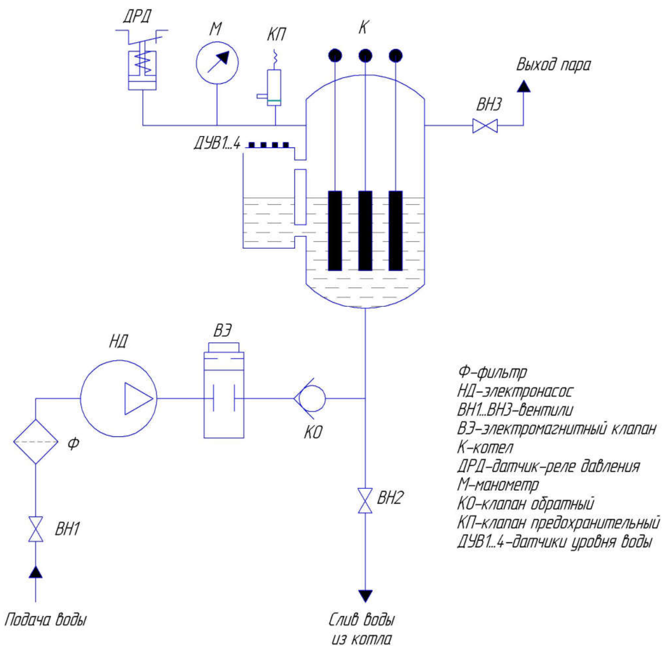
Рис.6 Паровая схема (одно- и двухступенчатых парогенераторов )
