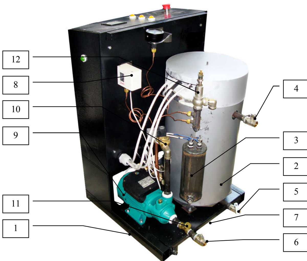
Рис.2 Внешний вид парогенератора (одно- и двухступенчатых )
