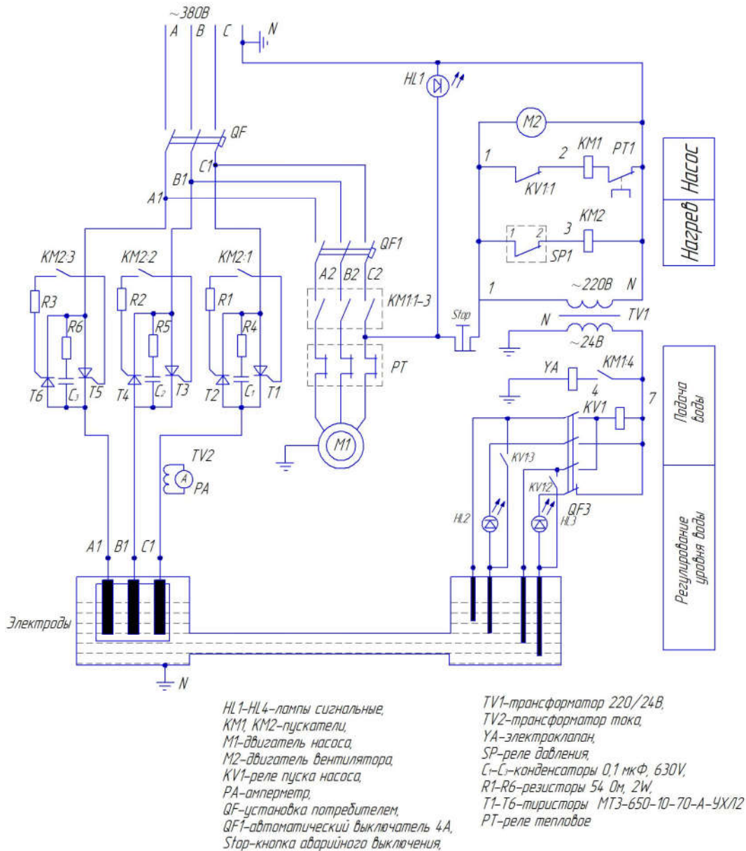
Рис.11 Схема электрическая двухступенчатых парогенераторов (управление тока нагрева тиристорами)
