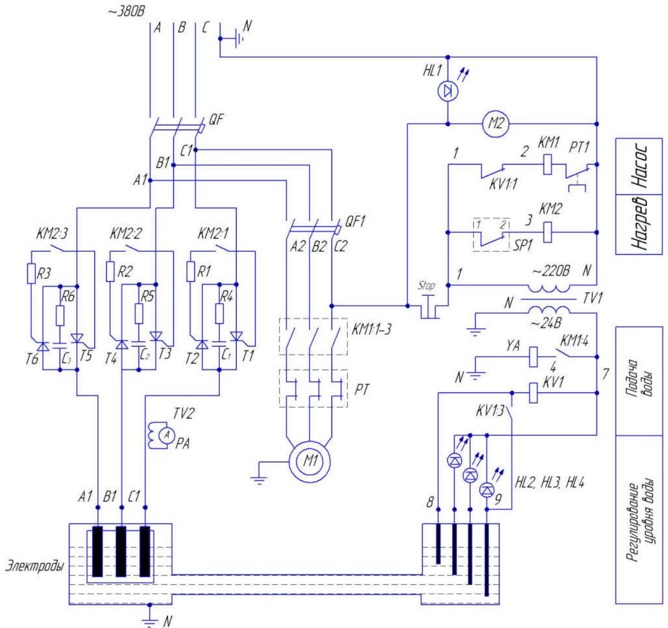
Рис.9 Схема электрическая (управление тока нагрева тиристорными модулями)
