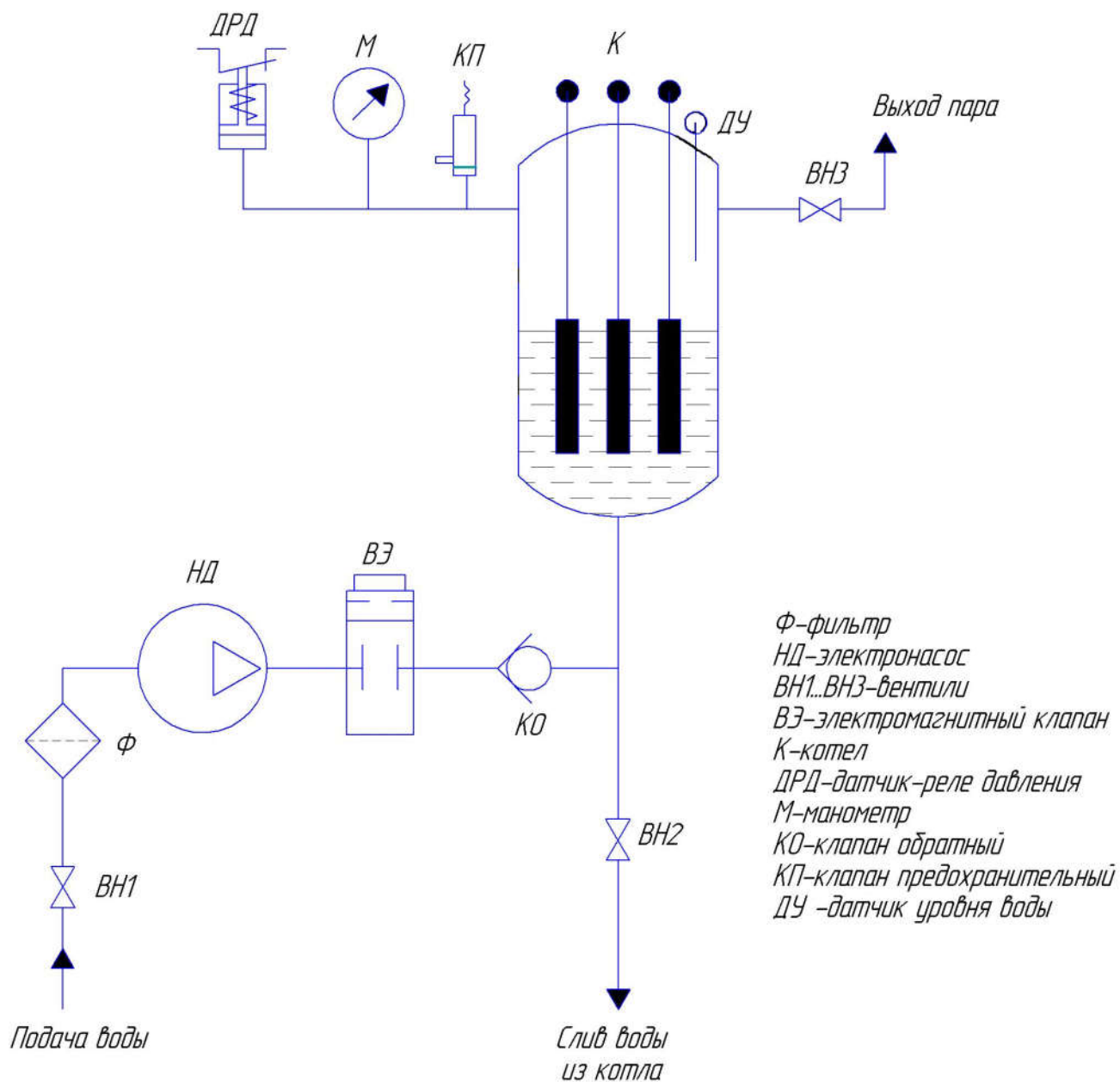
Рис.7 Паровая схема (парогенераторов с плавной регулировкой )
