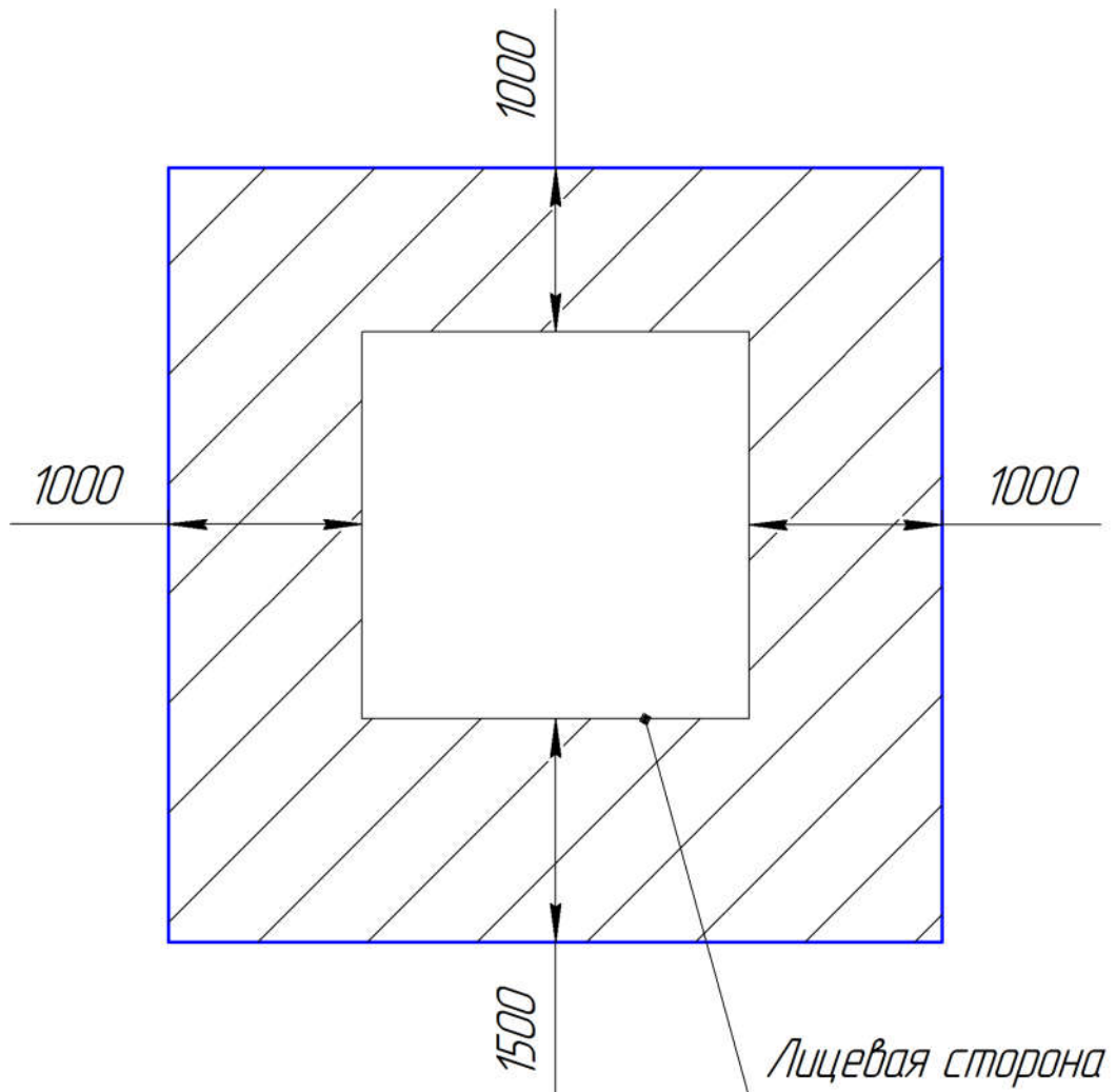
Рис. 15 Размеры рабочих зон для монтажа
