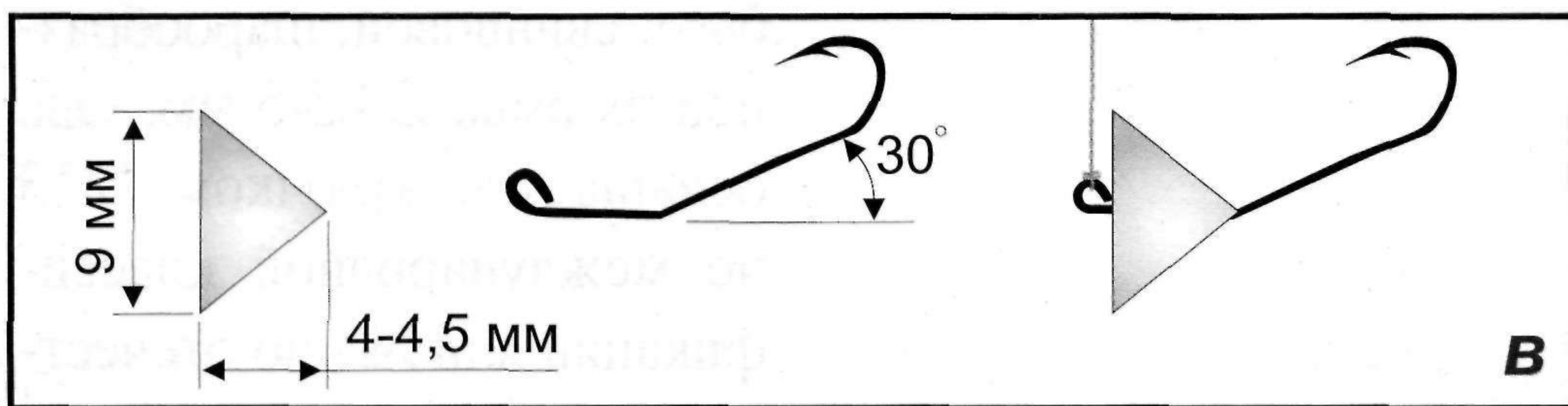
1.Мормышки для ловли карася: а – шарообразная для ловли в толще воды; б – донная, цилиндрическая; в – с лепестком из жести для ловли со дна.
