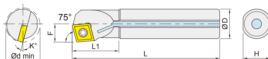
Coolant steel shank-right shown 中心出水鋼柄 右向示意圖
