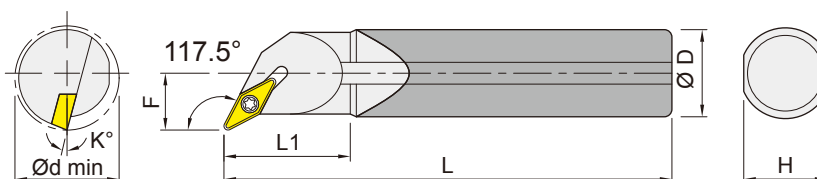
Carbide shank-right shown 鎢鋼柄 右向示意圖
