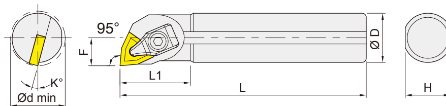
Steel shank-right shown 鋼柄 右向示意圖
