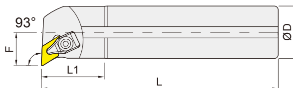
Steel shank-right shown 鋼柄 右向示意圖
