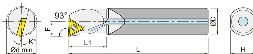
Coolant carbide shank-right shown 中心出水鎢鋼柄 右向示意圖
