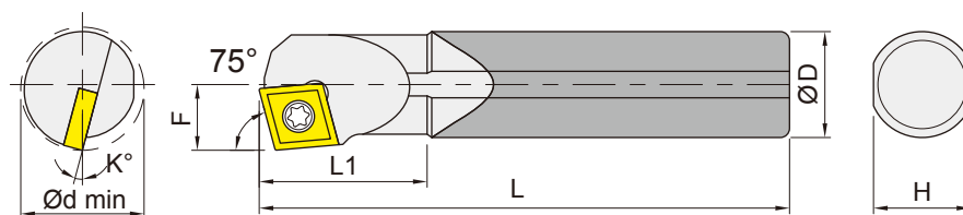
Carbide shank-right shown 鎢鋼柄 右向示意圖
