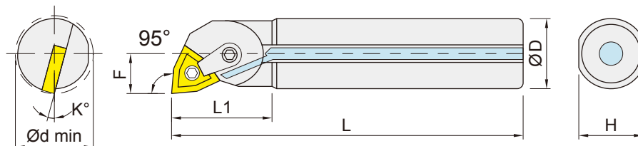
Coolant steel shank-right shown 中心出水鋼柄 右向示意圖
