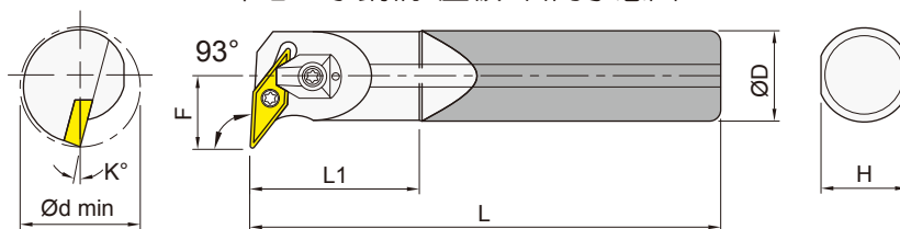
Carbide shank+clamp-right shown 鎢鋼柄+壓板 右向示意圖
