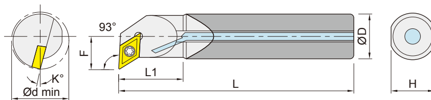
Coolant carbide shank-right shown 中心出水鎢鋼柄 右向示意圖
