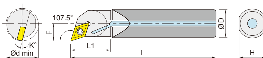
Coolant carbide shank-right shown 中心出水鎢鋼柄 右向示意圖
