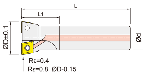
Coolant steel shank 中心出水鋼柄 示意圖
