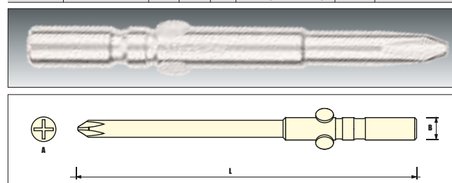
Биты одинарные PH 5 мм электро
