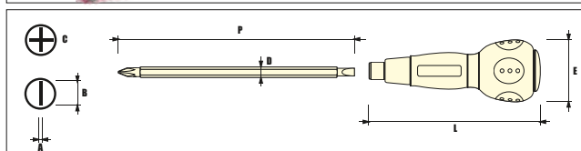
Отвертки со сменными наконечниками, диэлектрическая ручка
