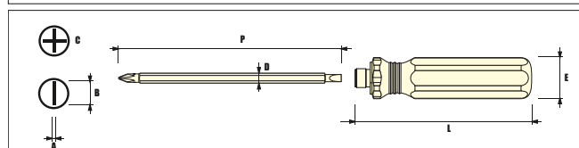
Отвертки со сменными наконечниками, цветная ручка
