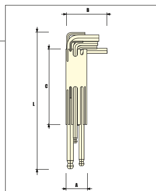
Шестигранные ключи со скругленным наконечником, хромированное покрытие - 9 шт.
