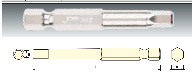
Биты одинарные шестигранные PH 6,35мм
