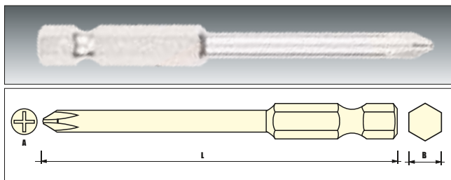
Биты одинарные PH электро
