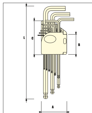
Шестигранные ключи со скругленным наконечником, вороненые - 9 шт.
