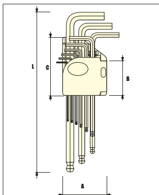
Шестигранные ключи со скругленным наконечником, зеркальное покрытие - 9 шт.
