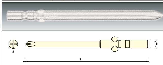
Биты одинарные PH 6мм электро
