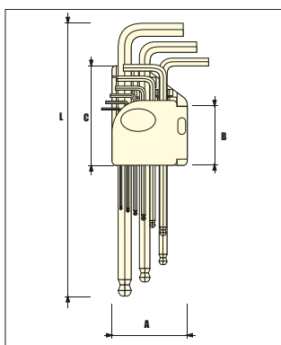
Шестигранные ключи со скругленным наконечником, хромированное покрытие (дюймы) - 9 шт.
