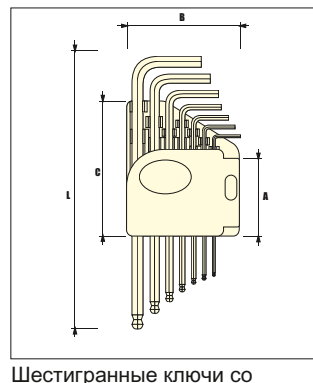
Шестигранные ключи со скругленным наконечником, матовый лак - 7 шт.
