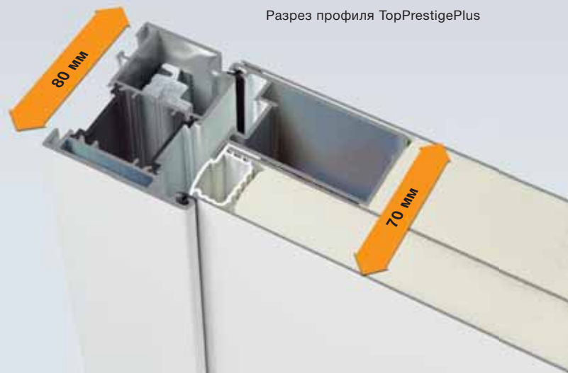
Разрез профиля TopPrestigePlus
