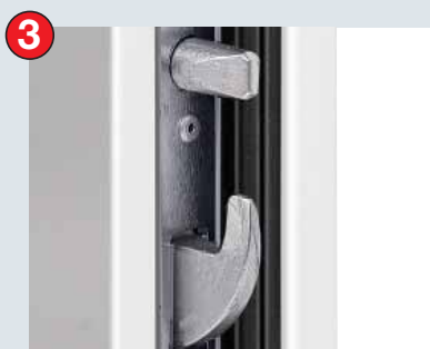
Поворотный ригель с запирающими штырями
