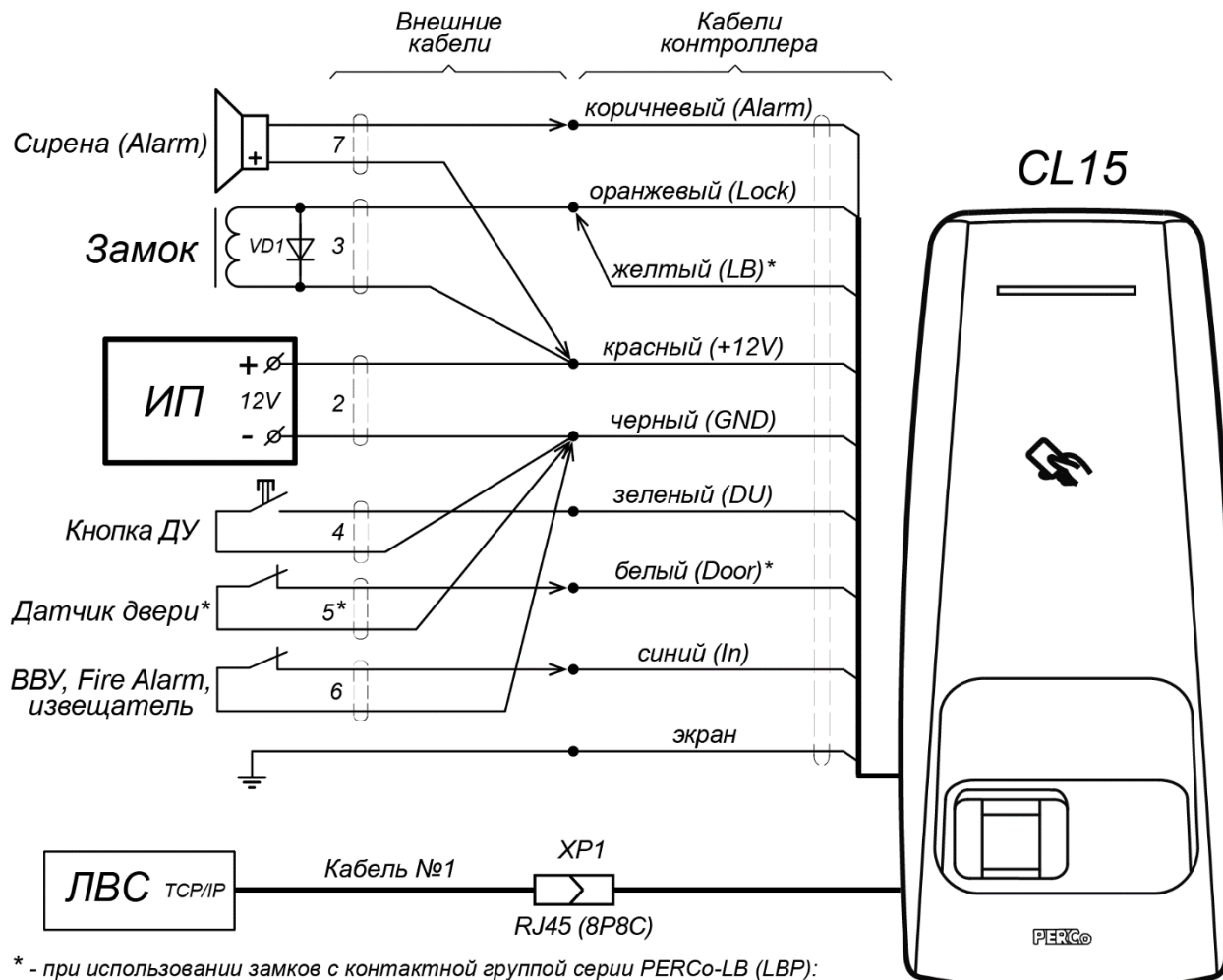
Рисунок 3. Схема подключений PERCo-CL15 для управления односторонним замком
