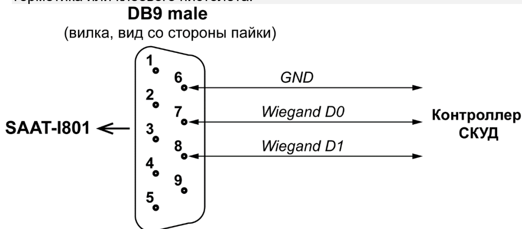
Рисунок 4. Подключение кабеля Wiegand
