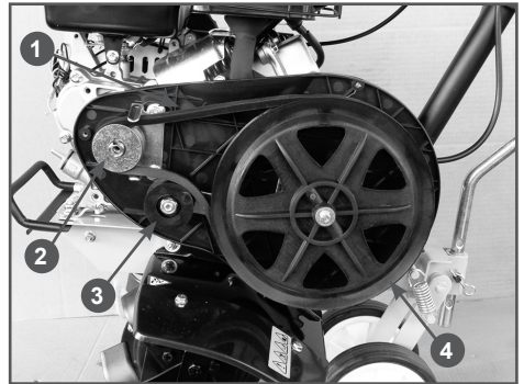
Рис. 23 Замена ремня привода
