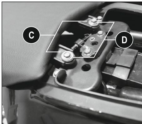
Крепежная скоба и отверстие в раме
