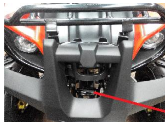
Номер двигателя
