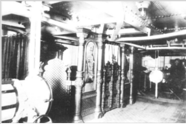
Помещение корабельной церкви на крейсере «Варяг». Справа и слева от алтаря видны торпедные аппараты
