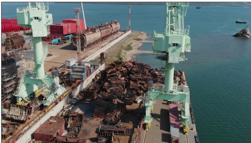
Разделочная площадка трехотсечных реакторных блоков в одноотсечные
