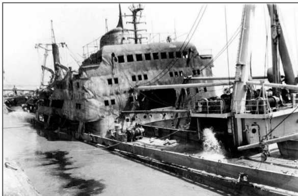
Извлеченное судно. Река Карнапхули
