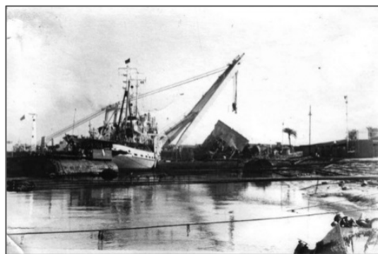
Судоподъемные работы в порту Читтагонг
