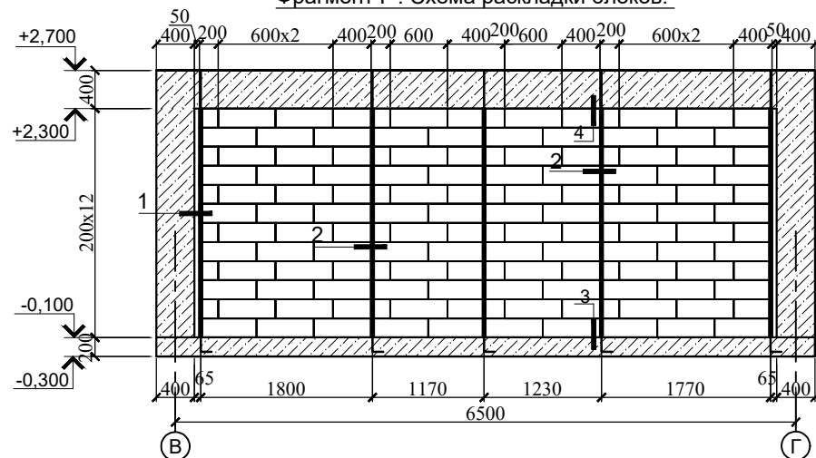
Фрагмент Г . Схема раскладки блоков.
