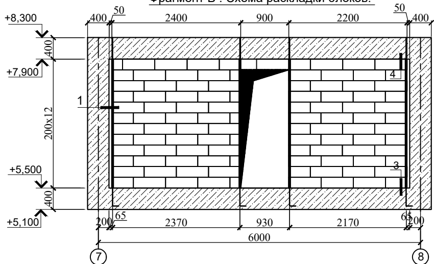
Фрагмент В . Схема раскладки блоков.
