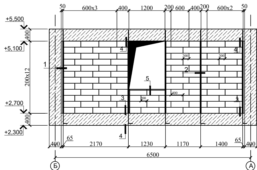
Фрагмент Г . Схема раскладки блоков.
