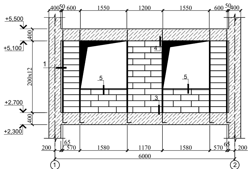
Фрагмент В . Схема раскладки блоков.
