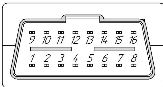
Рисунок 2.6 Нумерация выводов УМКа311
