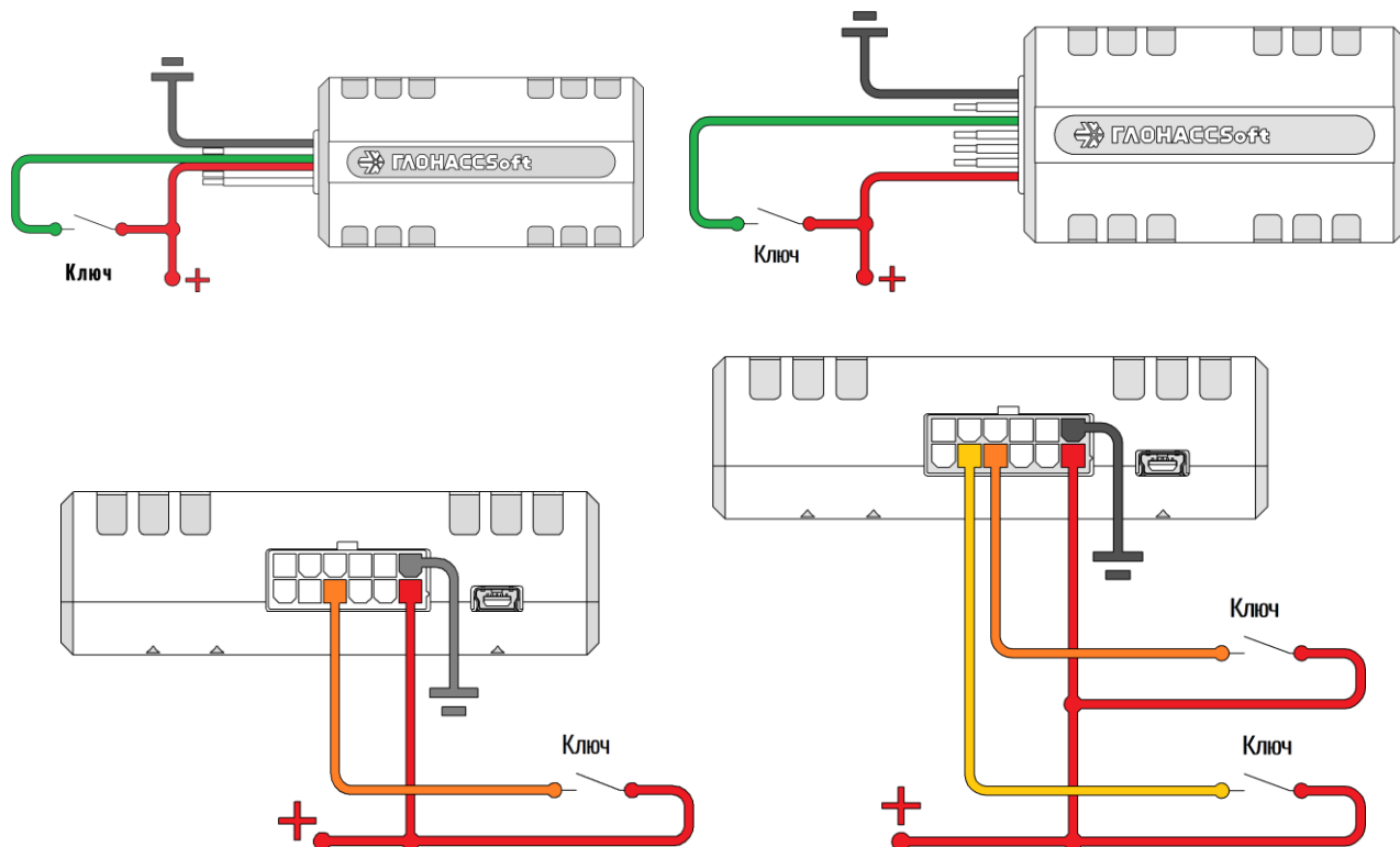
Рисунок 2.15 Подключение с подтяжкой к «-»
