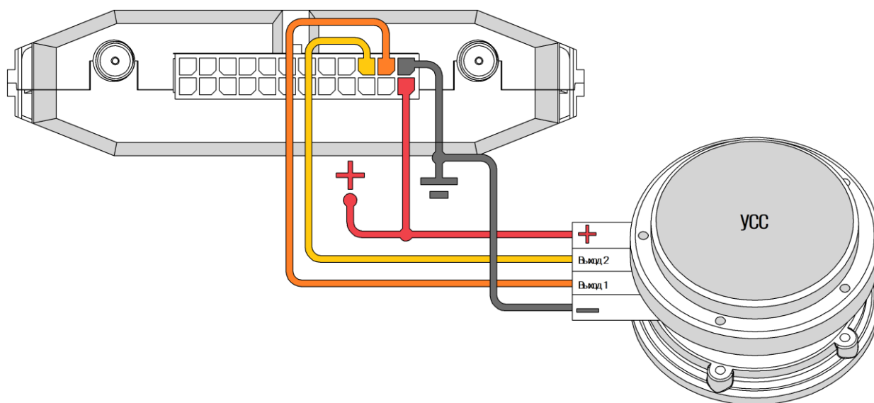
Рисунок 2.18 Пример подключения УСС
