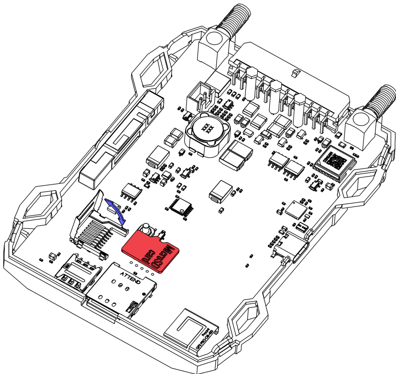
Рисунок 2.10 Установка microSD-карты
