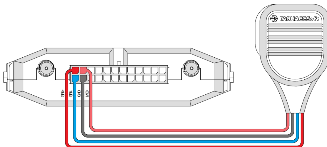
Рисунок 2.29 Схема подключения тангенты
