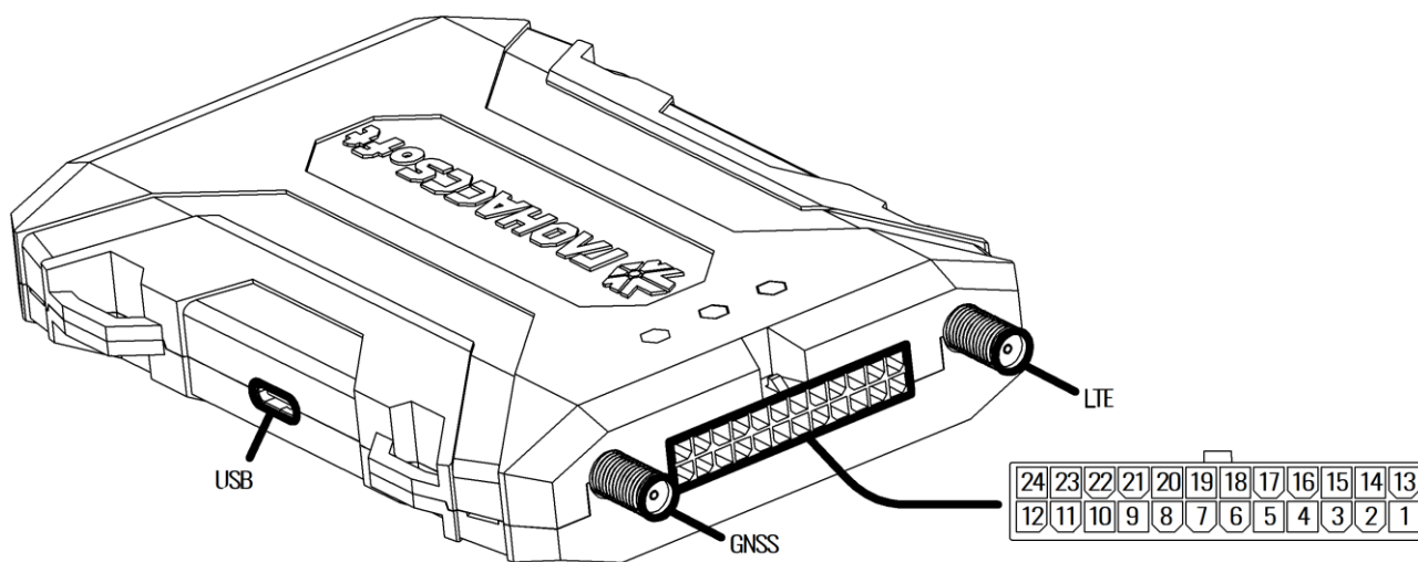
Рисунок 2.6 Нумерация выводов терминала
