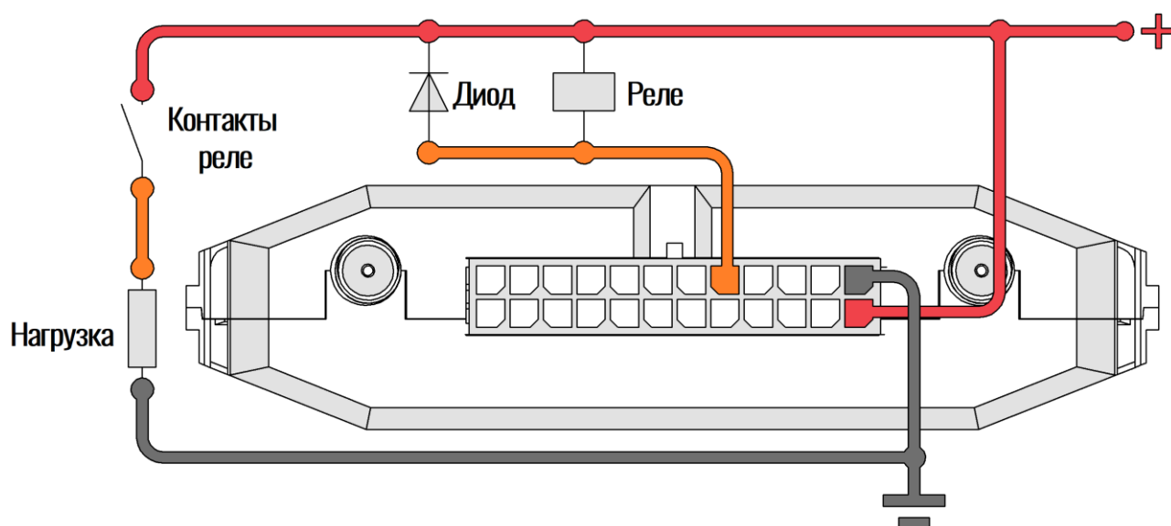
Рисунок 2.20 Подключение мощной нагрузки
