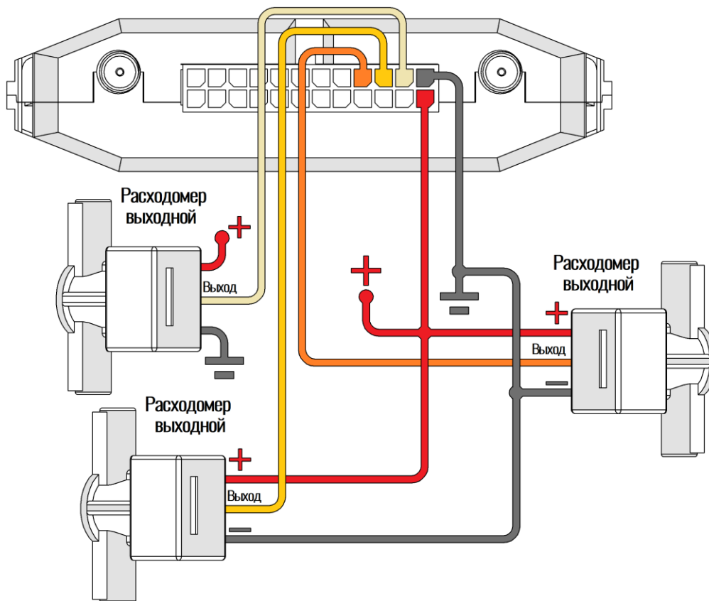
Рисунок 2.17 Пример подключения расходомеров в дифференциальном режиме
