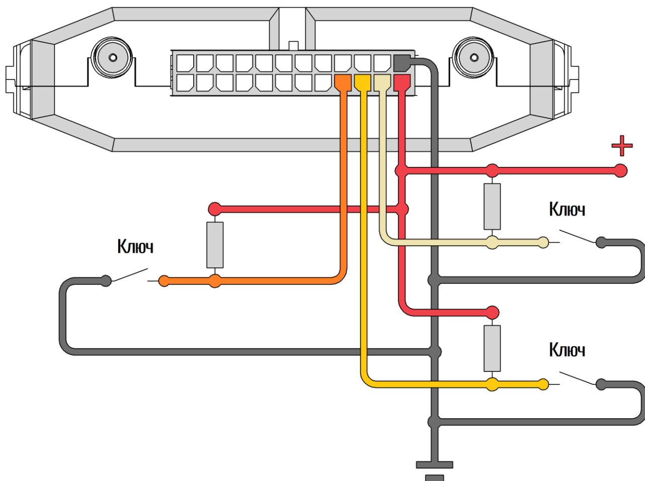
Рисунок 2.13 Подключение с подтяжкой к «+»
