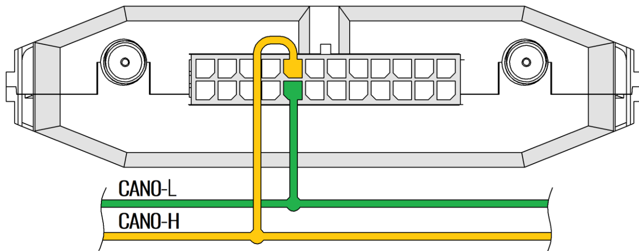
Рисунок 2.24 Подключение к шине CAN
