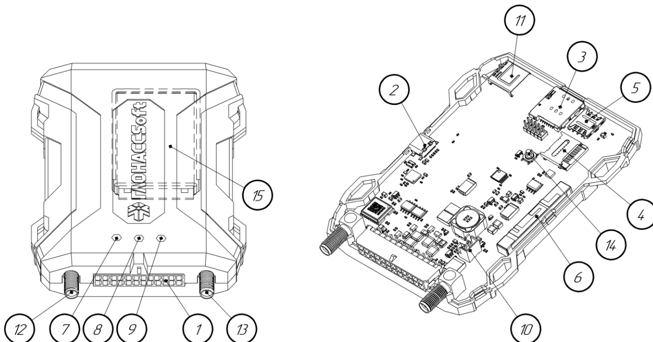
Рисунок 2.5 Основные элементы терминала
