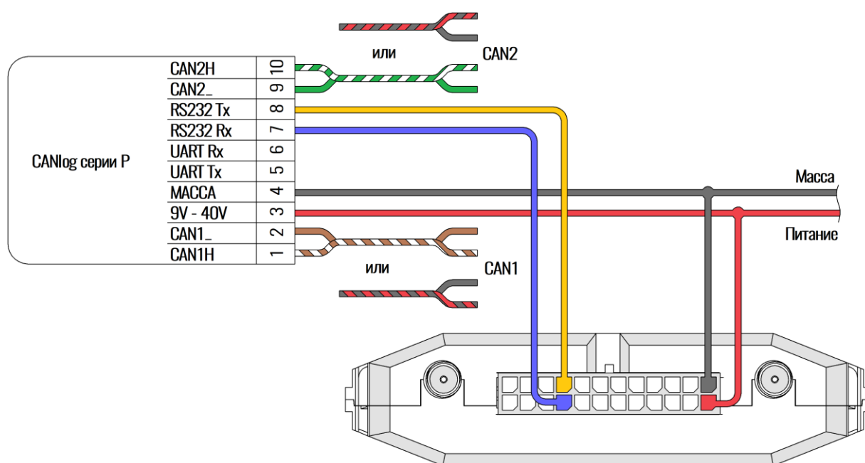
Рисунок 2.27 Подключение CAN-LOG по RS-232
