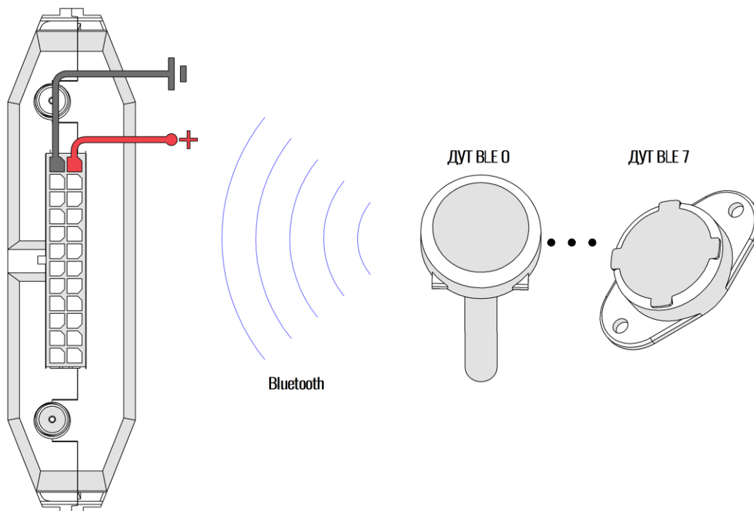
Рисунок 2.22 Подключение датчиков по BLE
