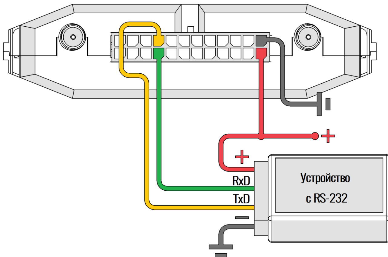
Рисунок 2.25 Подключение по интерфейсу RS-232
