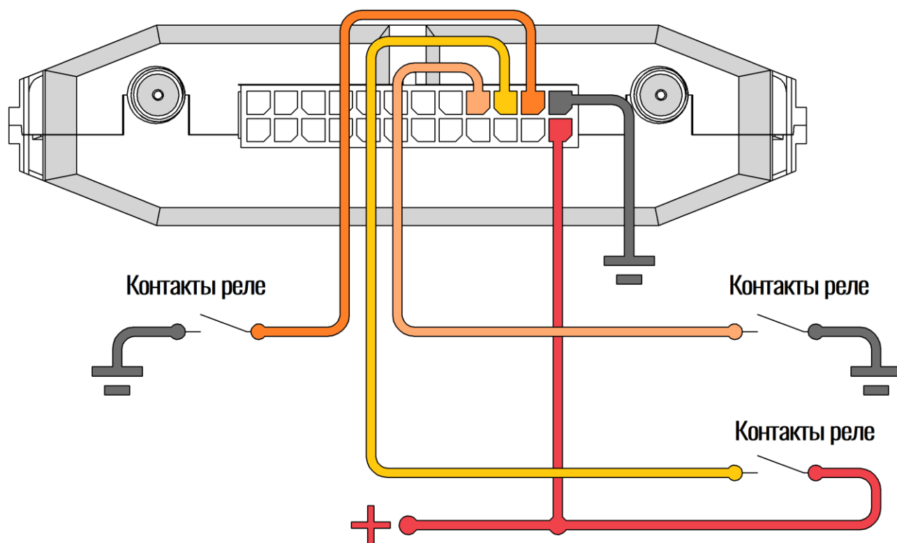
Рисунок 2.16 Варианты подключения дискретных датчиков
