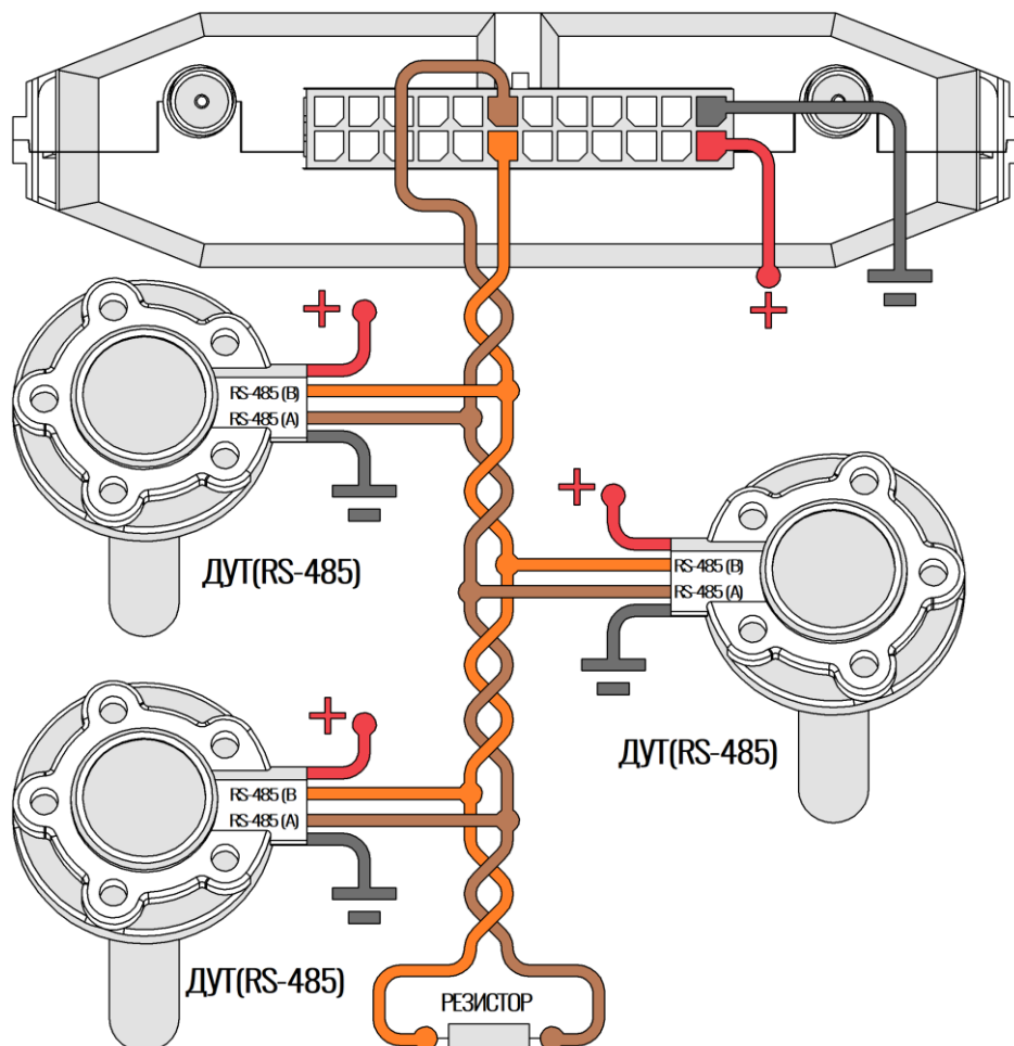
Рисунок 2.21 Подключение ДУТ по интерфейсу RS-485
