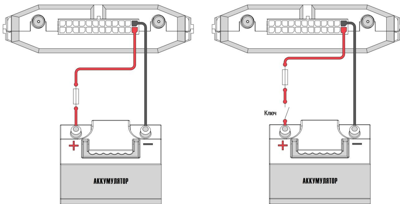
Рисунок 2.11 Подключение питания
