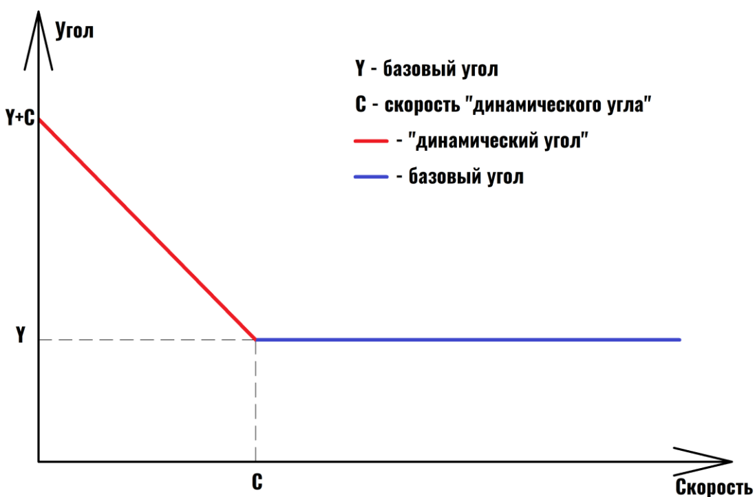
Рисунок 3.18 График зависимости динамического угла от скорости
