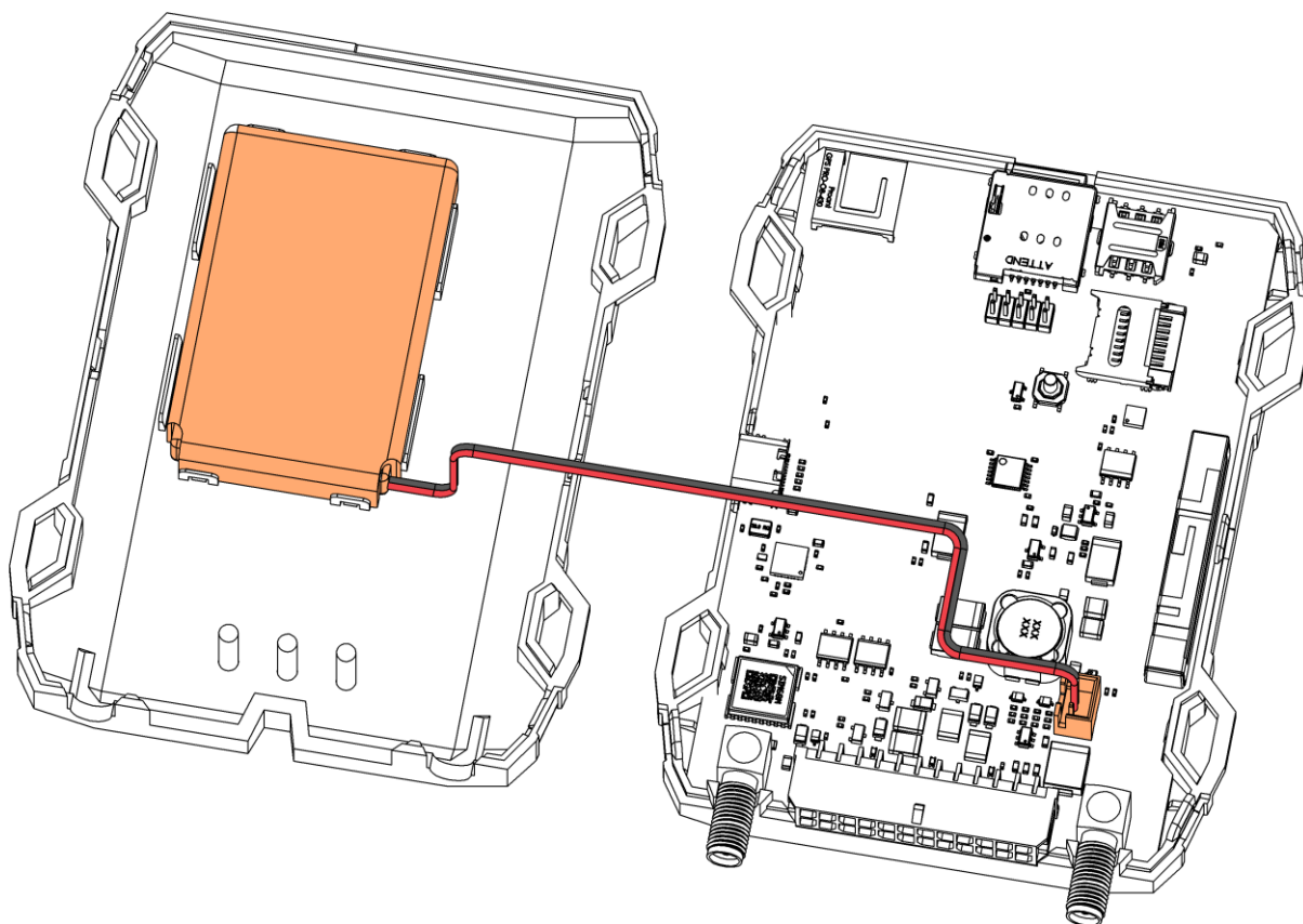
Рисунок 2.9 Установка аккумулятора
