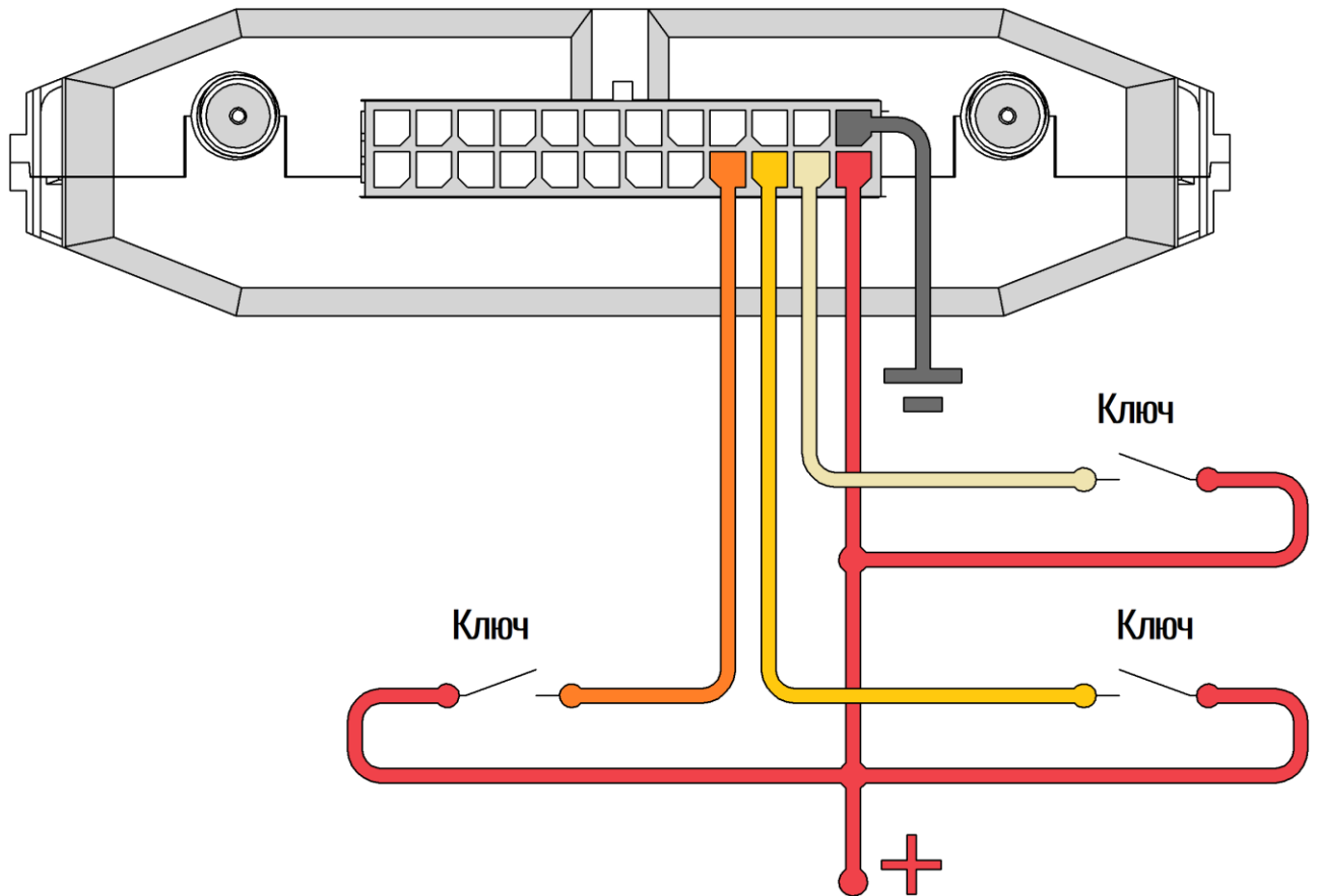
Рисунок 2.14 Подключение с подтяжкой к «-»
