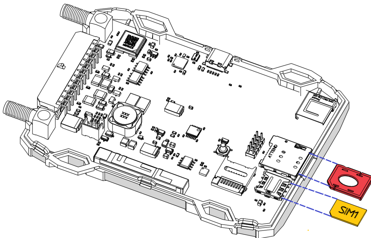
Рисунок 2.8 Установка SIM-карт
