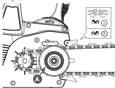
Рис. 3 Установка шины
