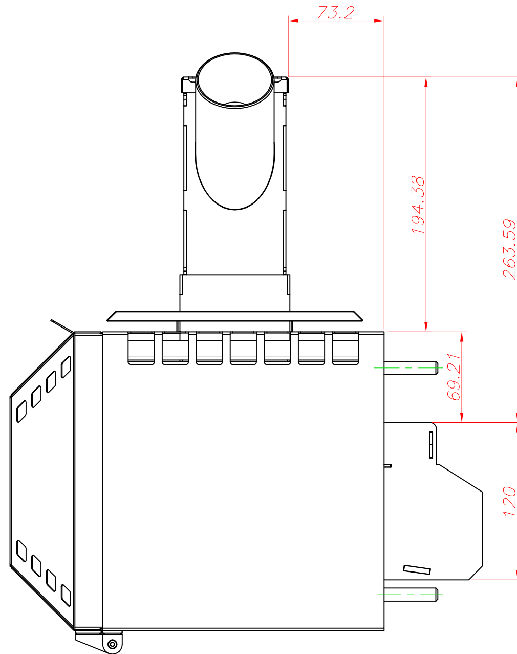
Горелка ГОР_20
