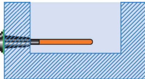
Пример: горизонтальное размещение нагревателей
