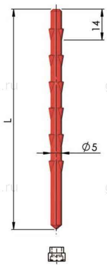
CERAMIC FERRULE: FER - 052 FOR STUD WELDING
