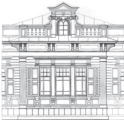
Рис. 18. Пример иркутского деревянного декора, имитирующего формы каменной архитектуры (ул. Декабрьских событий, 52). Чертеж фрагмента фасада. Источник: Калинина И. В., Красная Н. Н. Город и дерево. Архитектура и ремесло. — Иркутск: ООО Агентство «МайР», 2013. — 452 с., илл. С. 380.
