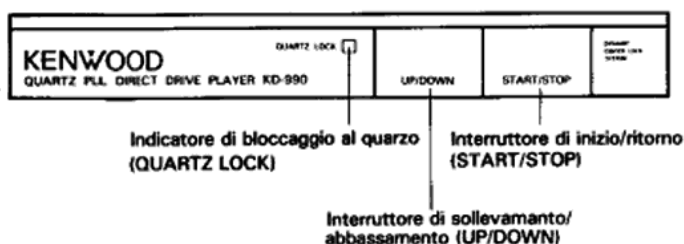
Fig. 18
