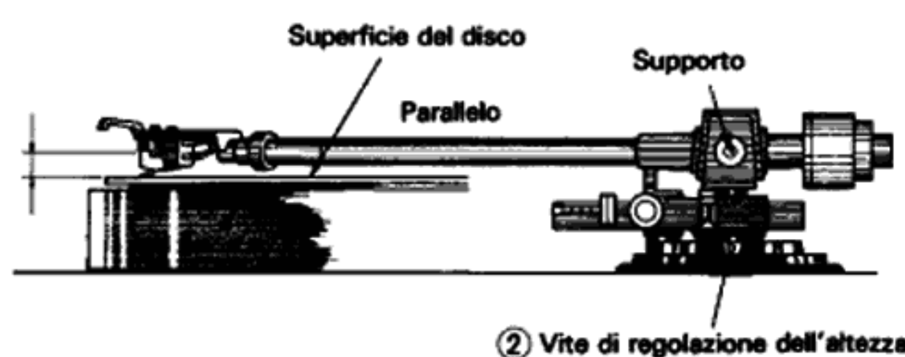
Fig. 16
