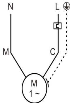
Схема подключения
