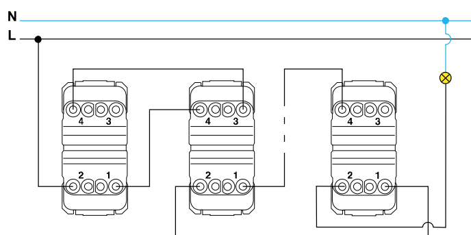
Два переключателя и необходимое количество перекрестных переключателей
