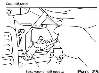
Замена (проверка) свечи зажигания
