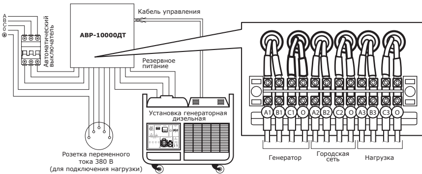
Рис. 23. Рекомендуемая схема подключения резерва АВР-10000ДТ
