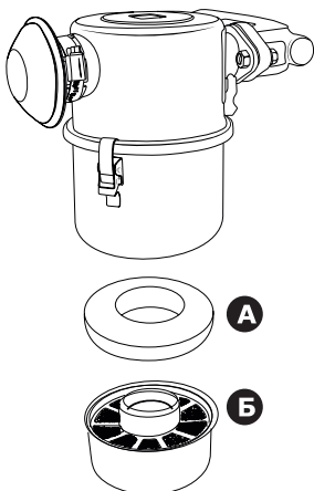
Рис. 27. Очистка воздушного фильтра для генераторов УГД-10000Е, УГД-100000ЕТ:
