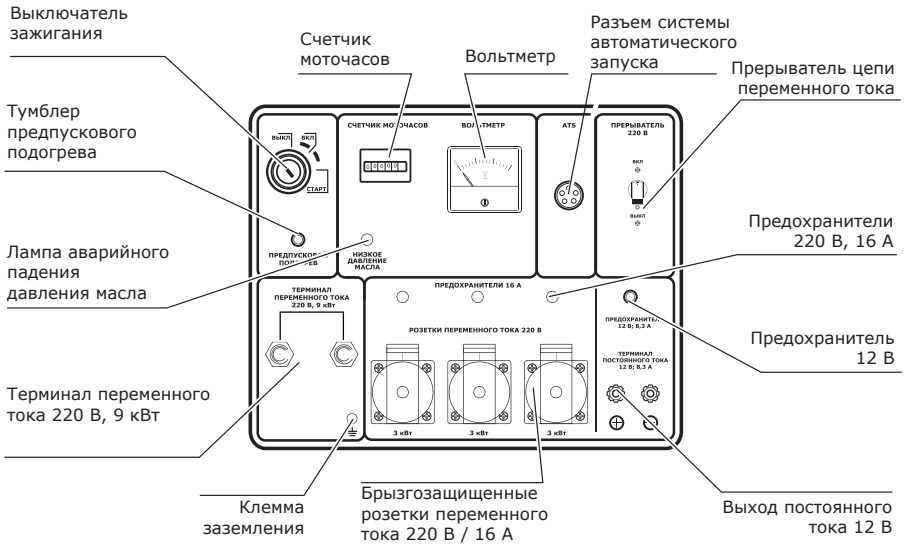
Рис. 4. Схема панели управления генератора УГД-1000Е
