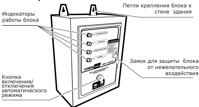
Рис. 19. Внешний вид блоков автоматического ввода резерва АВР-10000Д, АВР-10000ДТ (для моделей УГД-10000Е и УГД-10000ДТ соответственно).
