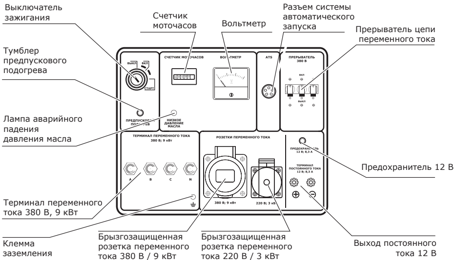
Рис. 5. Схема панели управления генератора УГД-1000ЕТ
