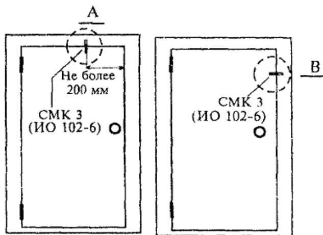
II Вариант установки (скрытая установка)
