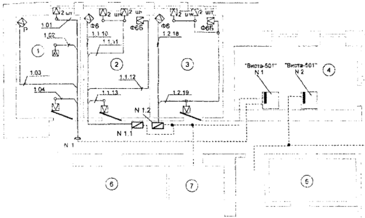
Рисунок 5 - Вариант выполнения схемы закладных
