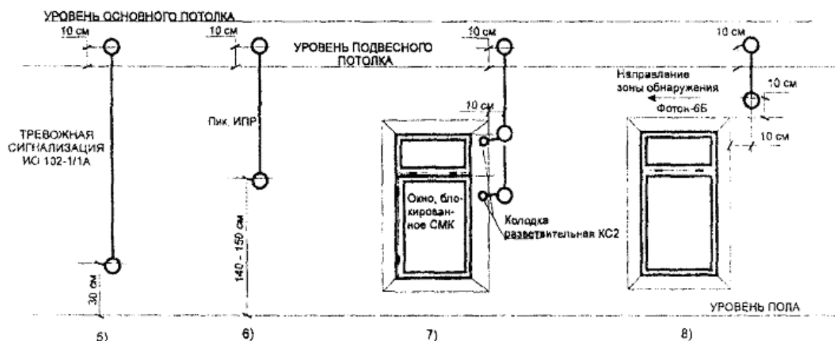
Рисунок 4 - Варианты расположения закладных для ТС ОПС в помещениях объекта
