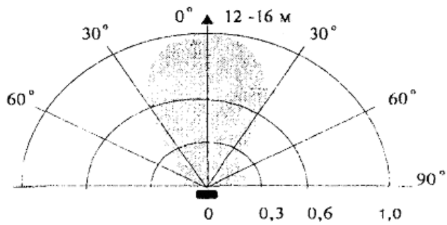
Рисунок 3 - Вариант блокировки объема помещения радиоволновым извещателем. (Размещение и схема подключения извещателя)
