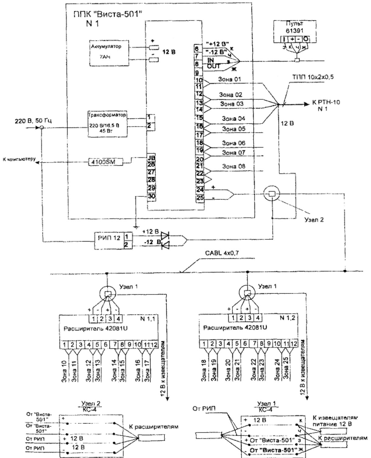
Рисунок 8 - Вариант выполнения электрической схемы соединений
