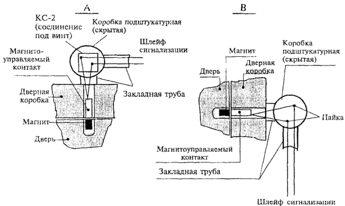
Рисунок 1 - Варианты установки магнитоконтактных извещателей на дверь
