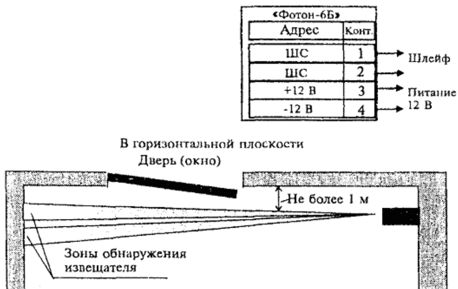
Рисунок 2 - Вариант блокировки двери (окна) на открывание и проникновение. (Размещение и схема подключения извещателей)
