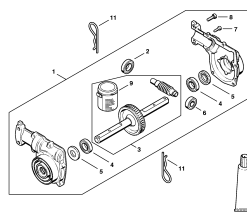
Передача
