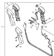
Рукоятка управления
