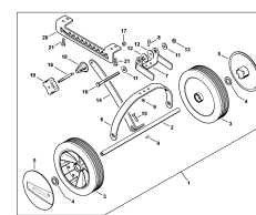
Комплект - Колёса
