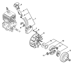
Система зажигания - Муфта
