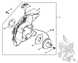
Пусковое устройство
