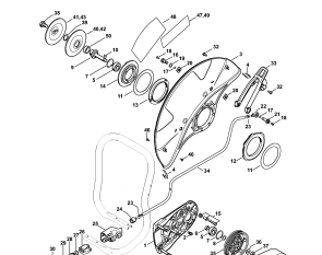
Подшипник с защитой С присоединением воды
