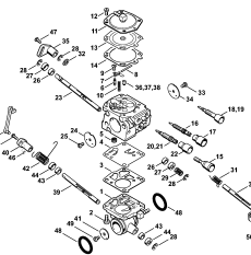
Карбюратор WJ-114, WJ-130
