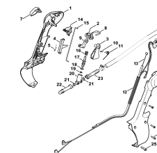
Рукоятка управления
