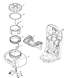
Опора - Резервуар
