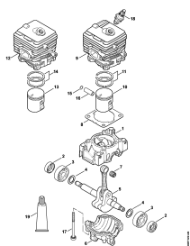
Картер - Цилиндр
