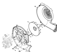
Корпус вентилятора, Крыльчатка вентилятора
