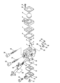
Карбюратор C1M-S244
