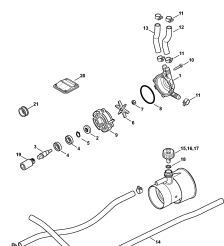
Нагнетательный насос
