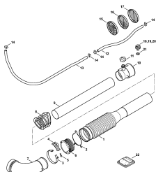
Гофрированный шланг - Пневматическая труба
