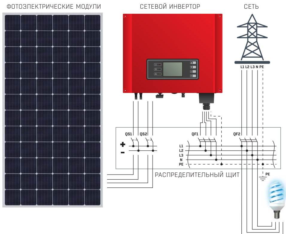
Блок-схема по подключению оборудования Системы С4-М
