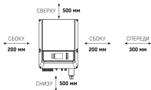
Рисунок 3.4.3 Расстояния до места установки инвертора
