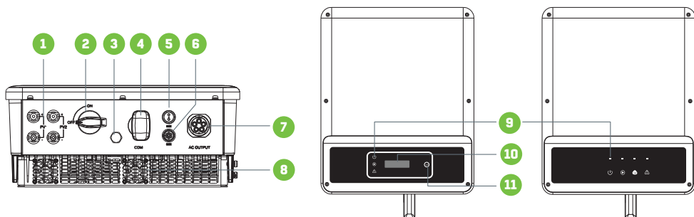
Рисунок 2.3.1 Схема инвертора
