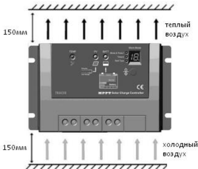
Рис.2. Установка контроллера
