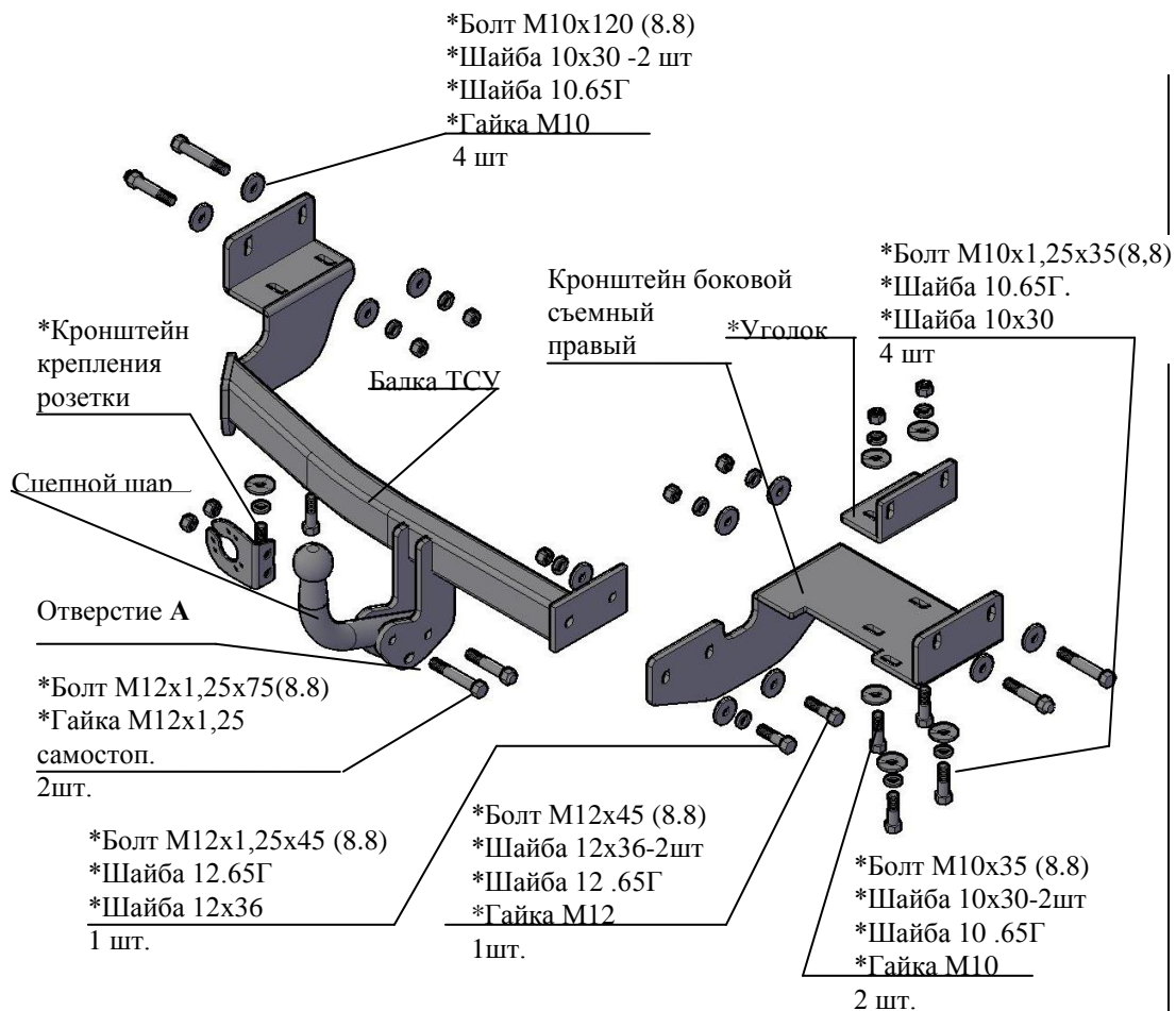
Рис.1 Тягово-сцепное устройство 7360
