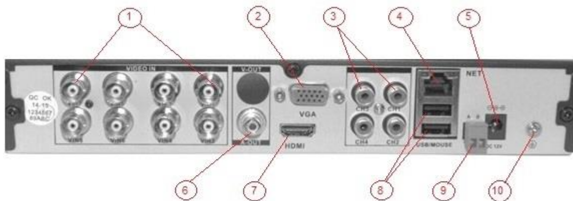
Задняя панель CTV-HD908A LITE
