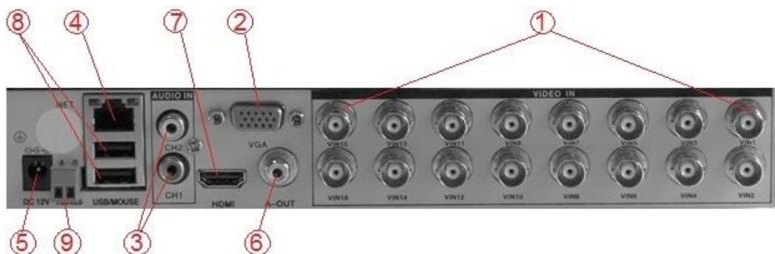
Задняя панель CTV-HD916A LITE
